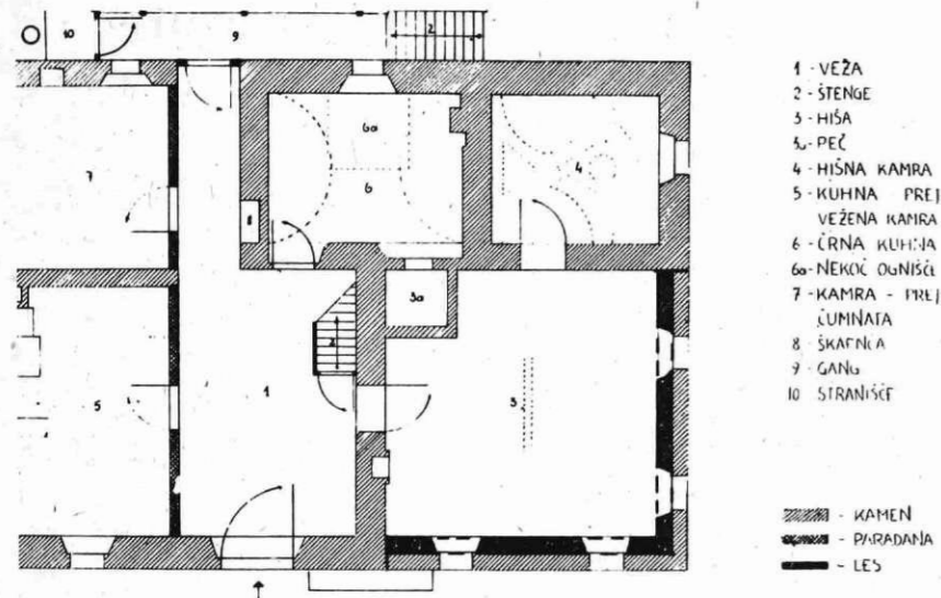
Tloris pritličja Liznekove hiše; temnejše so označeni prezidani deli zidov (prej leseni)
