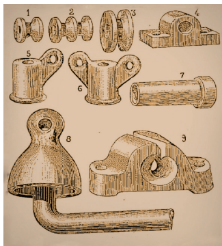
1885 Porcelain electrical insulators (La physique moderne : l'électricité dans la maison, É.Hospitalier)
