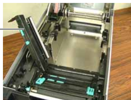
Obere Sensoreinheit
