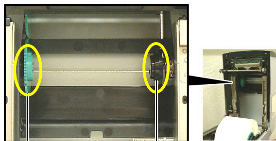
Farbbandaufnahme (Vorratsseite)
