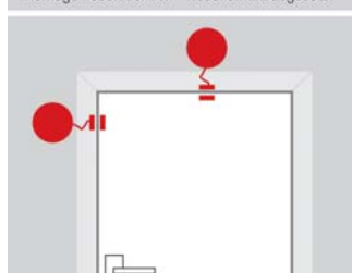
Montage neben der Tür – Reedkontakt abgesetzt
