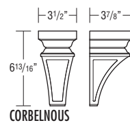
PLAIN NOUVEAU SMALL CORBEL R•26
