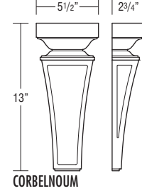
PLAIN NOUVEAU MEDIUM CORBEL R•26
