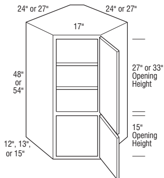
DW302424D L or R - DW362727D L or R
