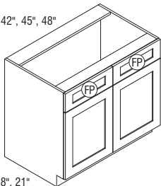
VSB3934 _- VSB4834 _- CS Vertical divider
