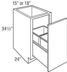
BWB15FH2 BWB18FH2
