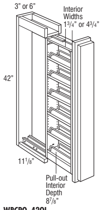
WBCPO_420L
