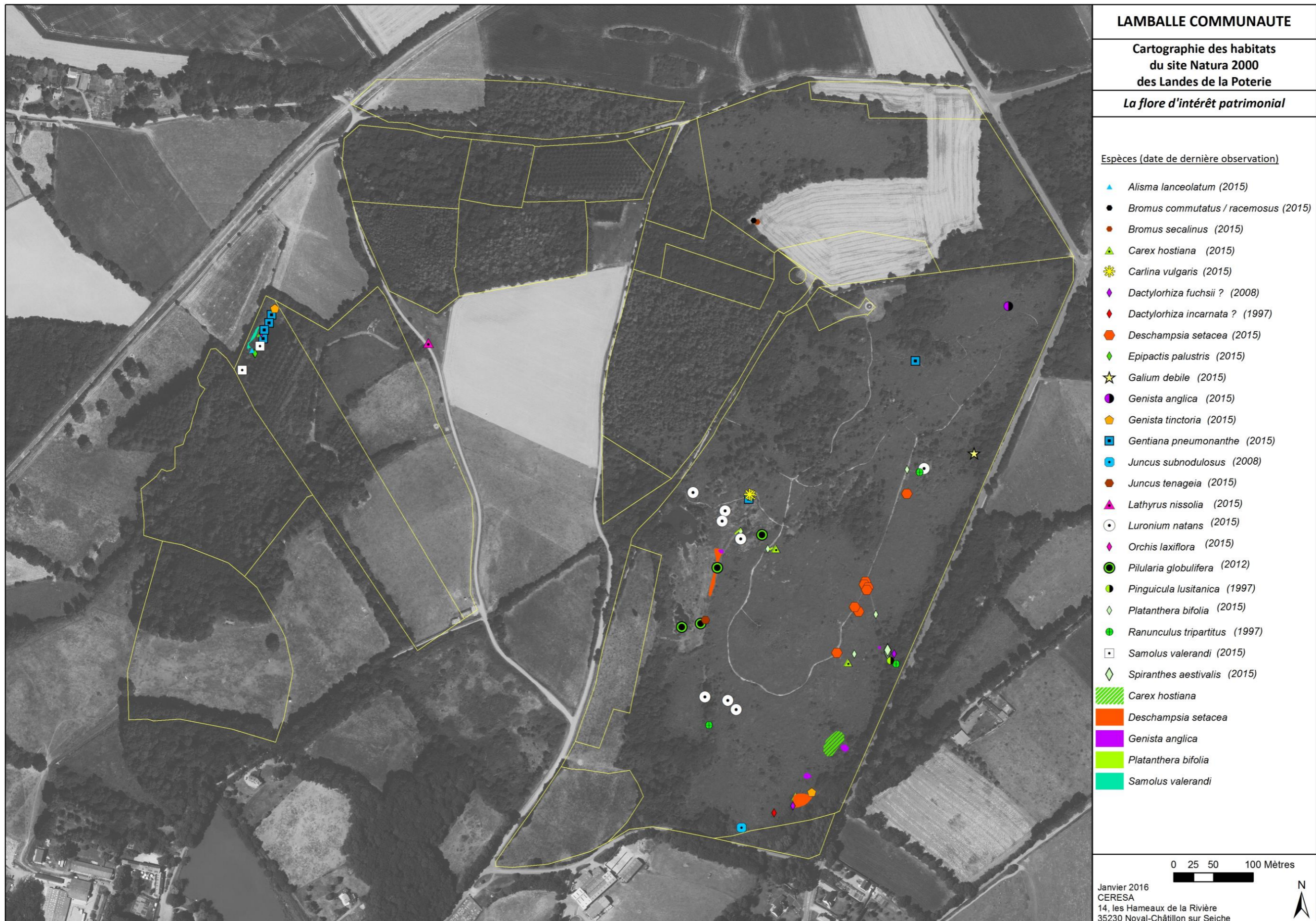
Carte 14 : Localisation de la flore d'intérêt patrimonial
