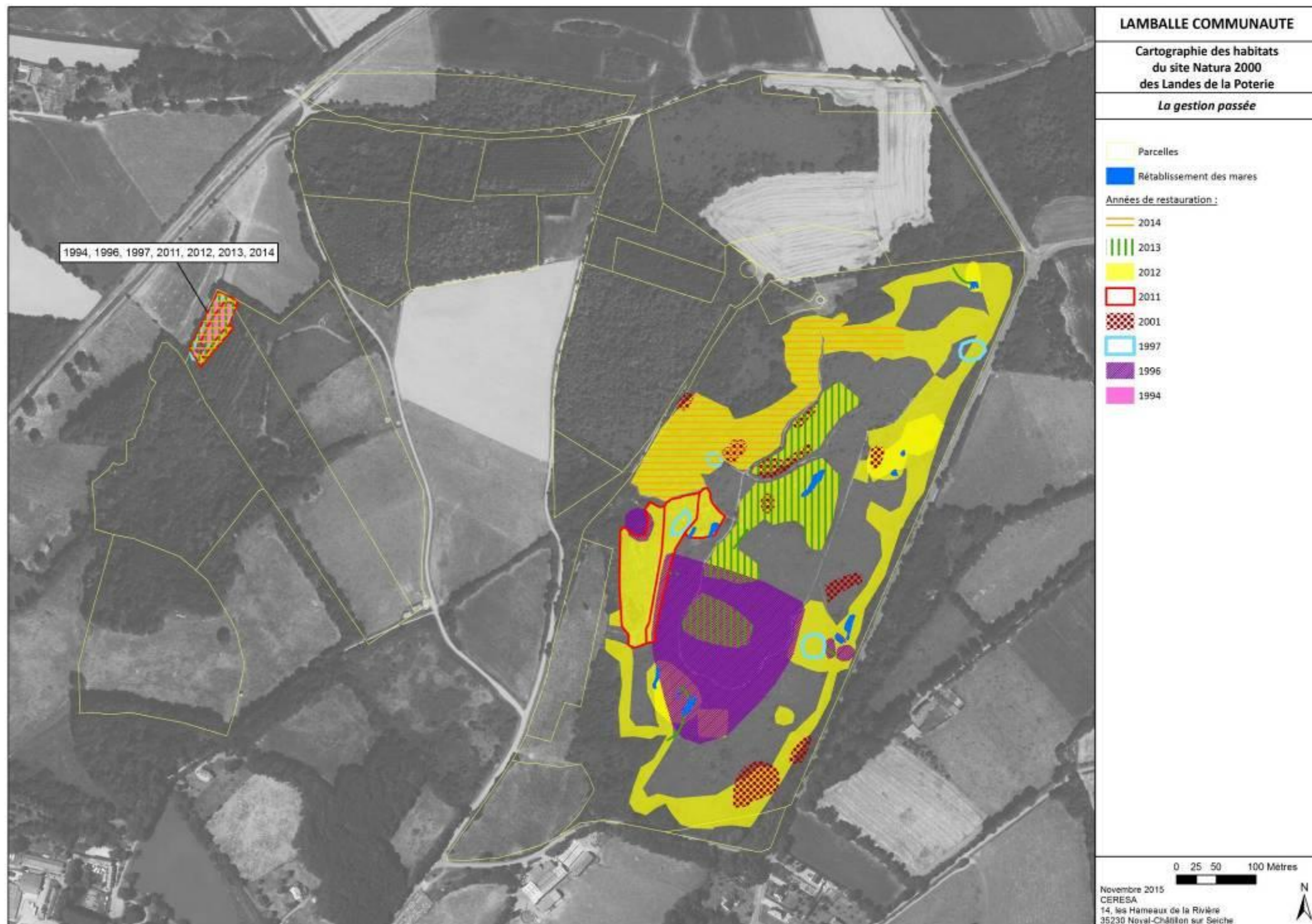
Carte 10 : La gestion passée des habitats naturels
