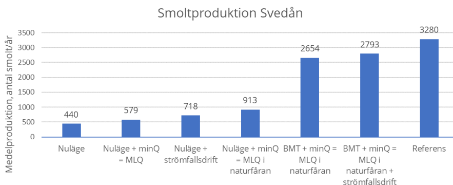
Figur 3: Figuren visar smoltproduktionsberäkningar vid olika åtgärdsscenario i delområdet.
