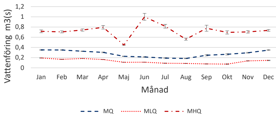
Figur 2. Stationskorrigerad vattenföring i Holmån baserat på modellerade dygnsvärden från SMHI:s vattenwebb mellan åren 2010–2021. I figuren framgår MLQ, MQ och MHQ (felstaplar anger P-varians).
