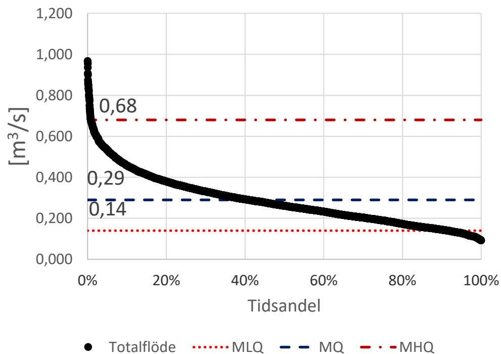
Figur 3. Varaktighetskurva för mätstationen Holmån (3689) med MLQ, MQ och MHQ visat i kubik per sekund över en bestämd period (2004–2020).
