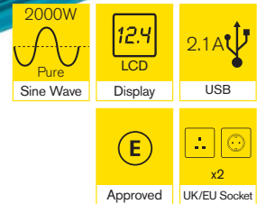
RINVP20/REINVP20 24V: RINVPB20/REINVPB20
