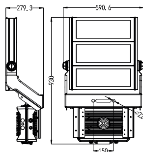
900W 590.6x930x279.3mm
