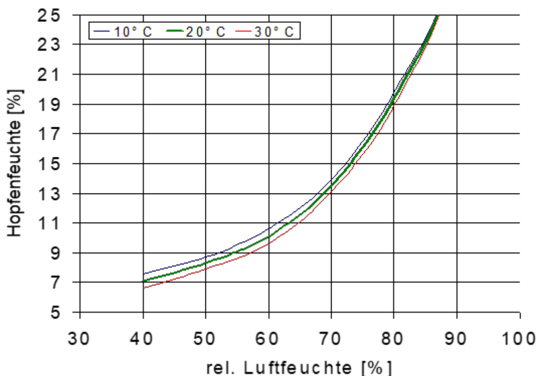
Abb.: Sorptionsisothermen von Hopfen
