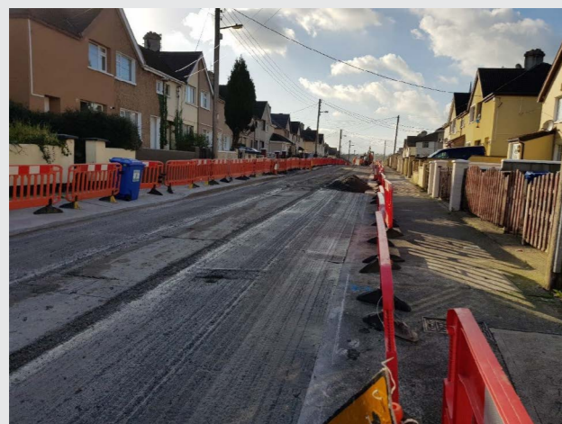
Oibreacha Bóthair ar siúl ag Sráid Uí Mhaoitúile, Garraí Eoin, Luimneach. Oibreacha a rinne Roadstone. Plánáil a dhéanamh ar an gcosán iomlán coincreíte atá ann. Dromchla Asfalt a chur ina ionad.
