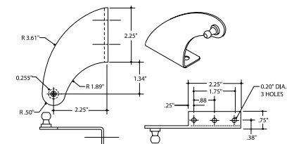
SL48
