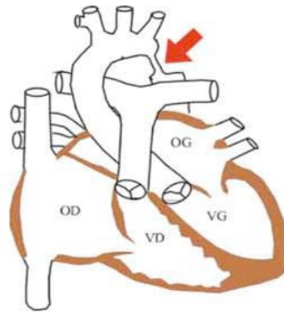
Figure n°3 : Coarctation de l'aorte
