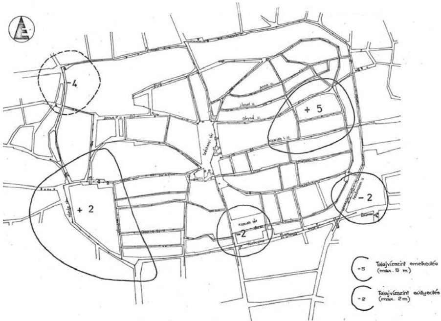
Talajvízszint-emelkedési- és süllyedési területek (szerk. Kaszás Ferenc)
