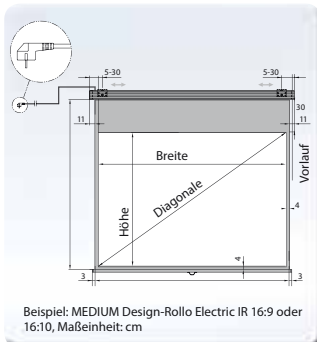
MEDIUM Design-Rollo Electric IR, Infrarotsteuerung mit Handsender und Netzstecker oder Wandbedienteil
