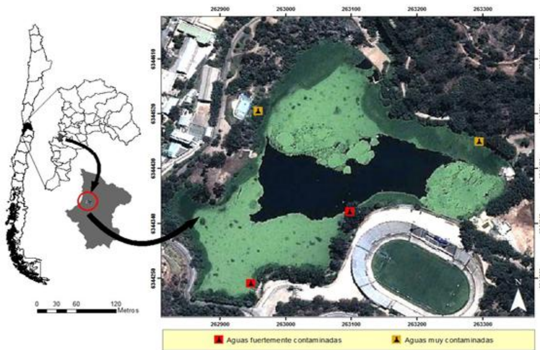
Figura 2: Calidad de aguas de la Laguna Sausalito según el Índice ChBMWP (modificado de Alba-Tercedor, 1996).
