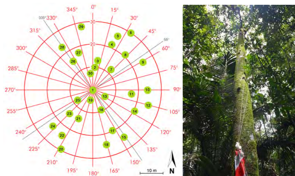
Bas fond (layon D) : L'aire d'échantillonnage correspond à l'aire de 30 x 40m utilisée pour la récolte des 20 Winkler du protocole Diadema. Les appâts thon/miel sont installés à 2 mètres du sol en matinée et récoltés l'après-midi sur 30 arbres dont la localisation exacte est mesurée au télémètre-boussole.
