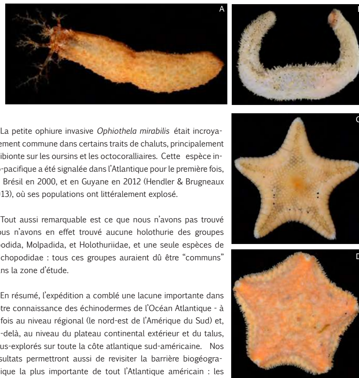
A. Euthyonacta n. sp. B. Mesothuria n. sp. C. Dipsacaster (?) n. sp. D. Porania aff. pulvillus
