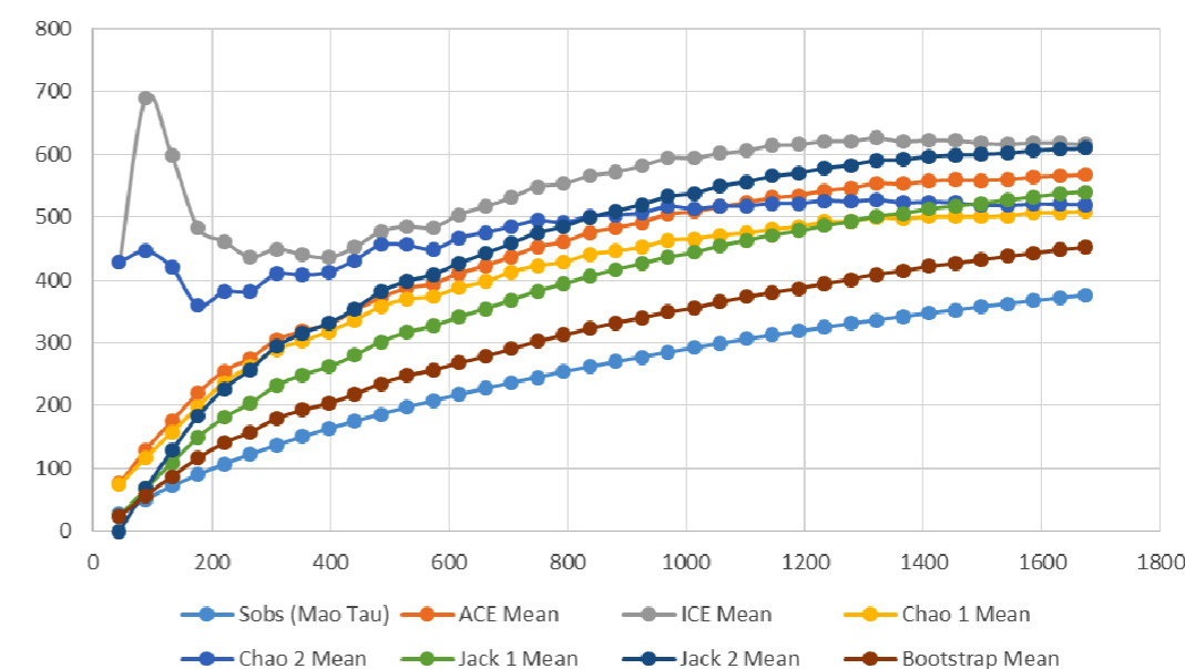
Figure 3. Courbe représentant l'accumulation des morpho espèces collectées en fonction du nombre d'individus collectés.
