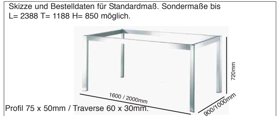
Tisch T50 Platte wird aufgelegt, Gestell jeweils einzeln. Traglast 120kg.
