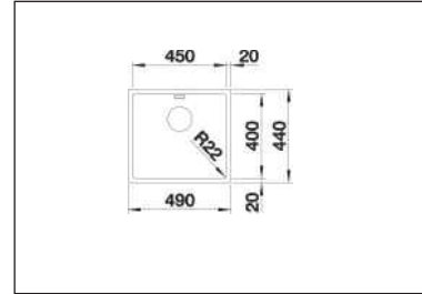
Unterbau-Becken 450-U inklusive Montagezubehör.
