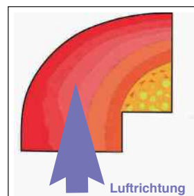
rot= hohe Luftgeschwindigkeit/Druck. gelb= kaum Druck, wenig Fluss, "Luftschatten".
