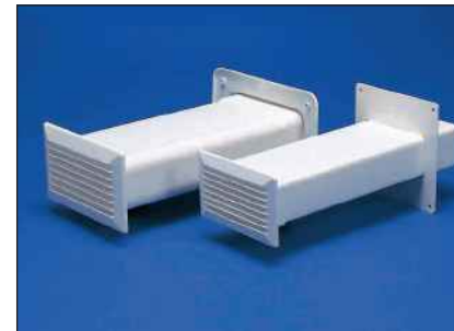
Flach-Mauerkasten bis Mauerstärke 500mm, 110 x 54mm, Gitter mit Rückstauklappe und Innenflansch. Durchbruch 116 x 60mm. Flansch aussen 145 x 90mm.
