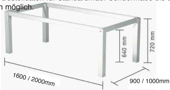
Tisch T120 Platte aufgelegt, Traverse ringsum leicht versetzt. Traglast 120kg.
