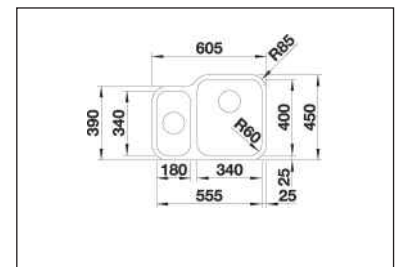
Unterbau-Becken Supra 340/180-U inklusive Montagezubehör.
