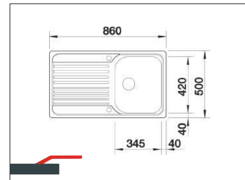
BlancoToga 45S Excenter Reversible Excenter-Spüle in interessantem Preis-/Leistungsverhältnis. Mit Ab-/Überlaufgarnitur.
