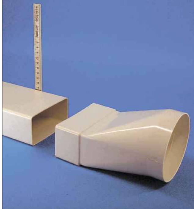
Flachrohr 100 Systemgrösse 110 x 54mm weiss
