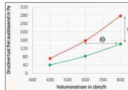
Rote Kurve: herkömmliches Umlenkstück Grüne Kurve: Kombi-Umlenkstück Optimairo
