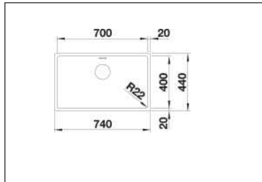
Unterbau-Becken 700-U inklusive Montagezubehör.
