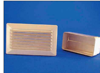
Flachgitter und Rückstauklappe Gitter für System 100 mit abnehmbarem Rückstauklappen-Kasten. Anschluss für Rohrverbinder. Durchbruch 116 x 60mm. Flansch aussen 135 x 75mm.
