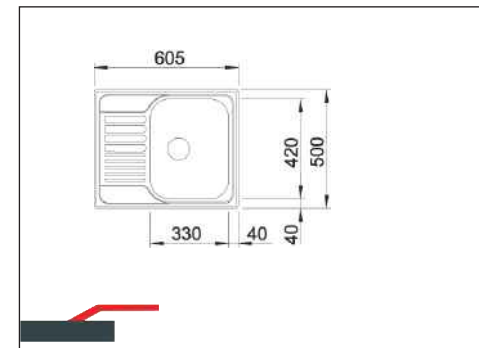
BlancoTipo 45 S Mini 605 x 500mm, reversibel, Siebkorbventil mit Ab-/Überlaufgarnitur. Ab 45er Schrank. Ausschnitt: 587 x 482mm.
