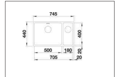
Unterbau-Becken 500/180-U inklusive Montagezubehör.
