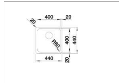
Supra 400 IF Flacheinbau sowie flächenbündig einbaubar.
