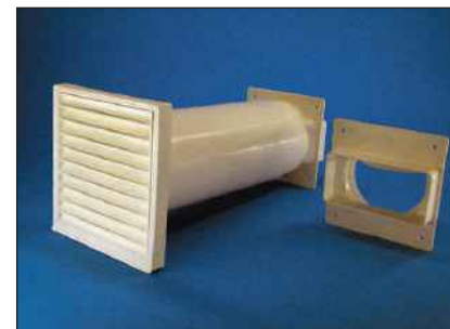
Rund-Mauerkasten mit Flachanschluss oder Rundanschluss. Flach= mit Muffe. Mit Rückstauklappe, teleskopierbar bis 45cm. Durchbruch D= 135mm. Flansch aussen 150 x 155mm.
