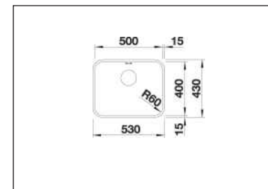
Unterbau-Becken Supra 500-U inklusive Montagezubehör.
