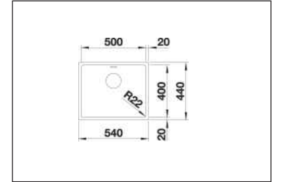
Unterbau-Becken 500-U inklusive Montagezubehör.
