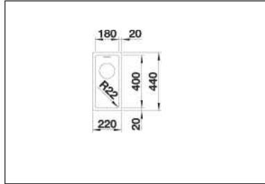
Unterbau-Becken 180-U inklusive Montagezubehör.
