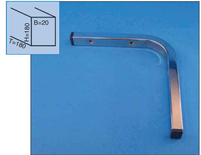
Wand- und Winkelkonsole 90° Rechteckrohr 20x15mm, Schenkel 180x180mm
