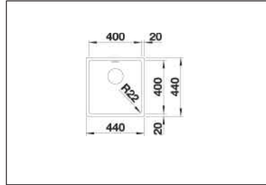
Unterbau-Becken 400-U inklusive Montagezubehör.
