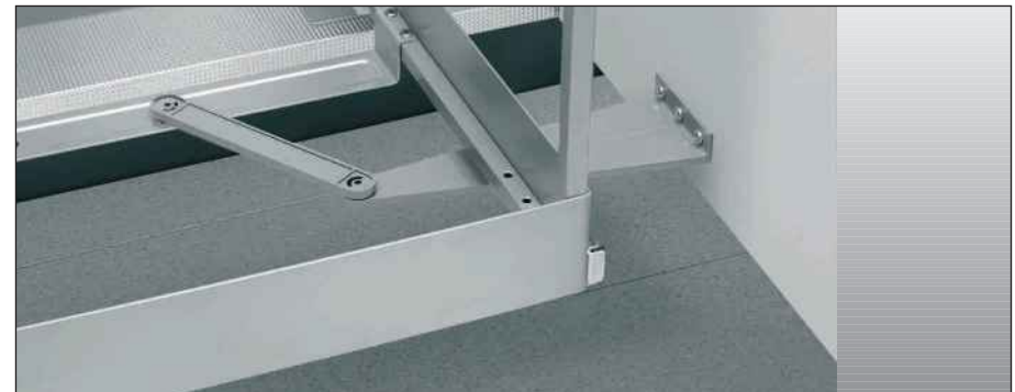
Hailo Raumspar-Tandem ab 60er Kompakte Bauweise - flach und kurz. Einfache Bodenmontage des Abfallsammlers mit zweifach- oder dreifach-Trennung. Kugelgeführter Vollauszug. Für Drehtürenschränke ab 60cm.
