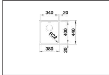
Unterbau-Becken 340-U inklusive Montagezubehör.
