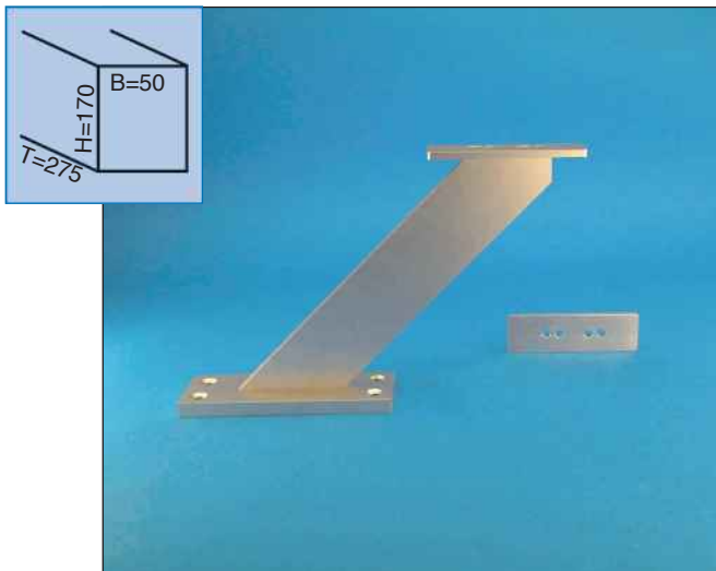
Schräg-Konsole Alu Mit Bohrschablone und Montagematerial. Maße: Höhe 170mm, Tiefe total 275mm, Länge obere Platte 140mm, Länge untere Platte 80mm, Plattenbreite unten 30mm und oben 50mm.
