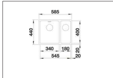
Unterbau-Becken 340/180-U inklusive Montagezubehör.
