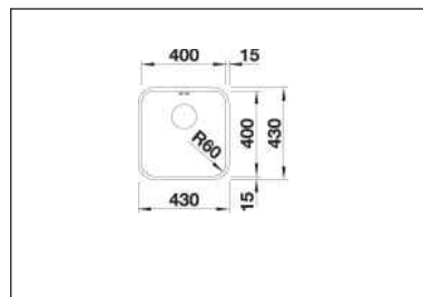
Unterbau-Becken Supra 400-U inklusive Montagezubehör.
