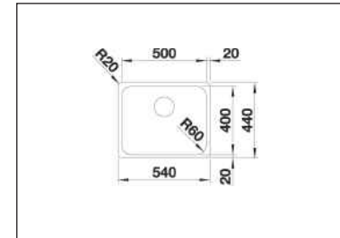
Supra 500 IF Flacheinbau sowie flächenbündig einbaubar.
