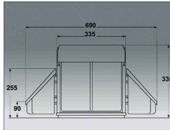
CornerBOY mit Seitenschalen (abnehmbar).
