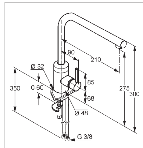
L-line Extravaganz und minimalistisches Design prägen dieses Produkt für die moderne, architektonische Küche. 360° Schwenkauslauf und auch für Niederdruck lieferbar.
