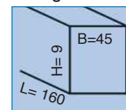
Oberbodenleuchte Flat , passend zur Unterbauleuchte (S. 81). Aus gebürstetem Edelstahl mit umlaufendem Lichtkranz. Zuleitung 1,8m, Leistung 1,5 Watt. Leuchtkopf 45x 45x 9mm. Länge überstehend 100mm. Geeignete Schalter ab Seite 110. Converter bei Einzelleuchten mitbestellen!
