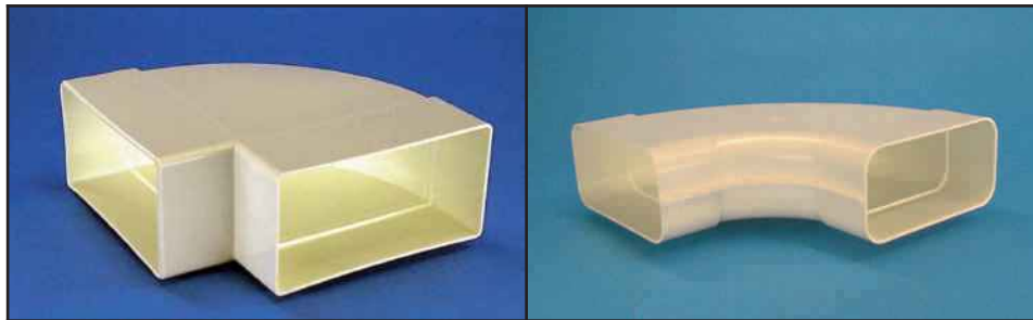
Die Bauform eines Formstückes wirkt sich wesentlich auf die Luftleistung aus.
