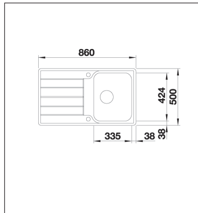
Blanco Classimo 45 S-IF Kompakte Excenter-Spüle mit grosszügig gestalteten Funktionsbereichen. Flacheinbau und flächenbündig. Ausschnitt 840 x 480.
