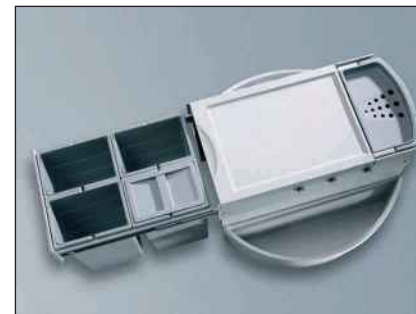
Rondo 2 - mit Funktionseimer, Biodeckel (ab 3fach), Kehrset und verschiebbaren Haken.
