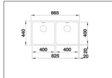
Unterbau-Becken 400/400-U inklusive Montagezubehör.
