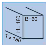
Nostalgie-Oberbodenleuchte mit weißem Mattglas-Kelch. Leuchtmittel LED Warmlicht 2,8 Watt.
