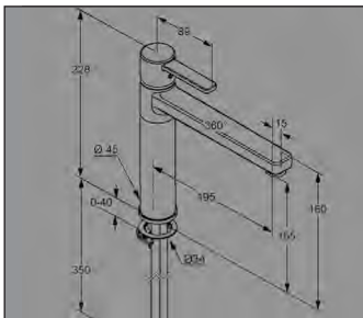
Kludi Zenta - auch in Edelstahl, schwarz und weiss ! Einhebelmischer in hohem, modernem Design. Auslauf, schwenkbar, mit flexiblen Anschlusschläuchen und Keramikkartusche mit Heisswasserbegrenzer.
