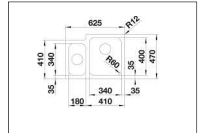
Supra 340/180 IF Flacheinbau sowie flächenbündig einbaubar.
