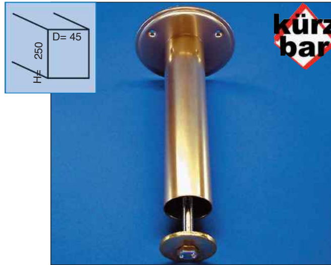
Maxi-Universalkonsole höhenvariabel zwischen 100mm und 250mm kürzen wir die Konsole millimetergenau. Platte oben D= 130mm.
