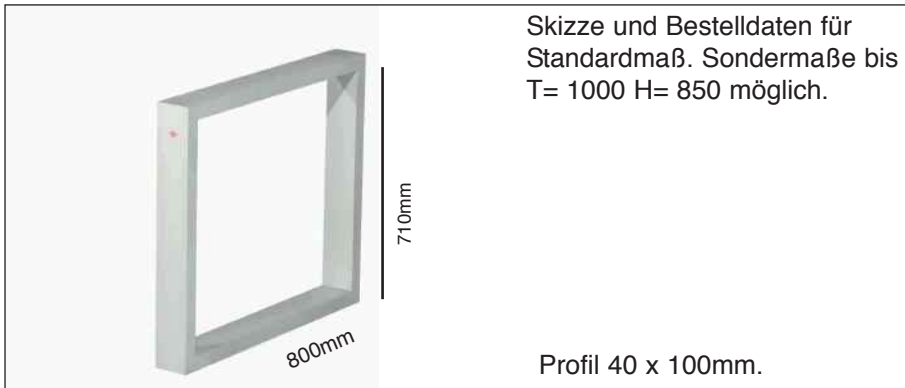
Tisch TG75 Platte wird aufgelegt, Gestell jeweils 1 Paar. Traglast 60kg.
