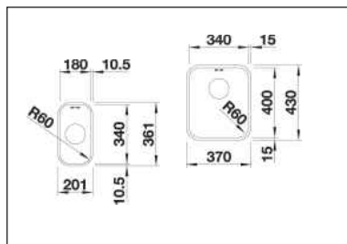
Unterbau-Becken Supra 180-U und 340-U
