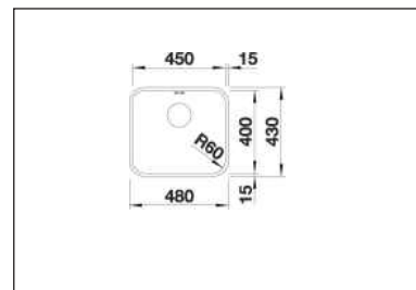
Unterbau-Becken Supra 450-U inklusive Montagezubehör.
