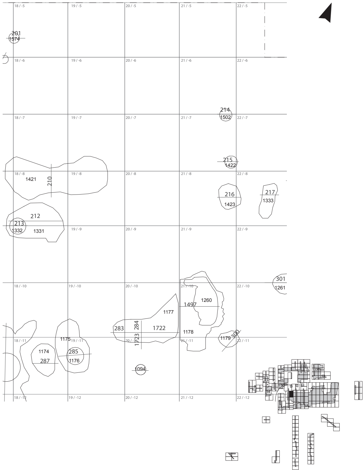
Planum LA 1 - Ausschnitt 44. M 1:125
