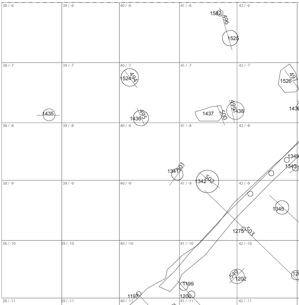
Planum LA 1 - Ausschnitt 73. M 1:125
