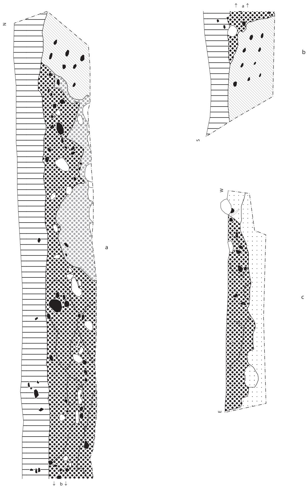
Befundtafel LA30_12 Profile Grabkammer 21 a u. b: Pr. 17 (Bef. 21; 21_7); c: Pr. 19 (Bef. 21_9). M 1:20.
