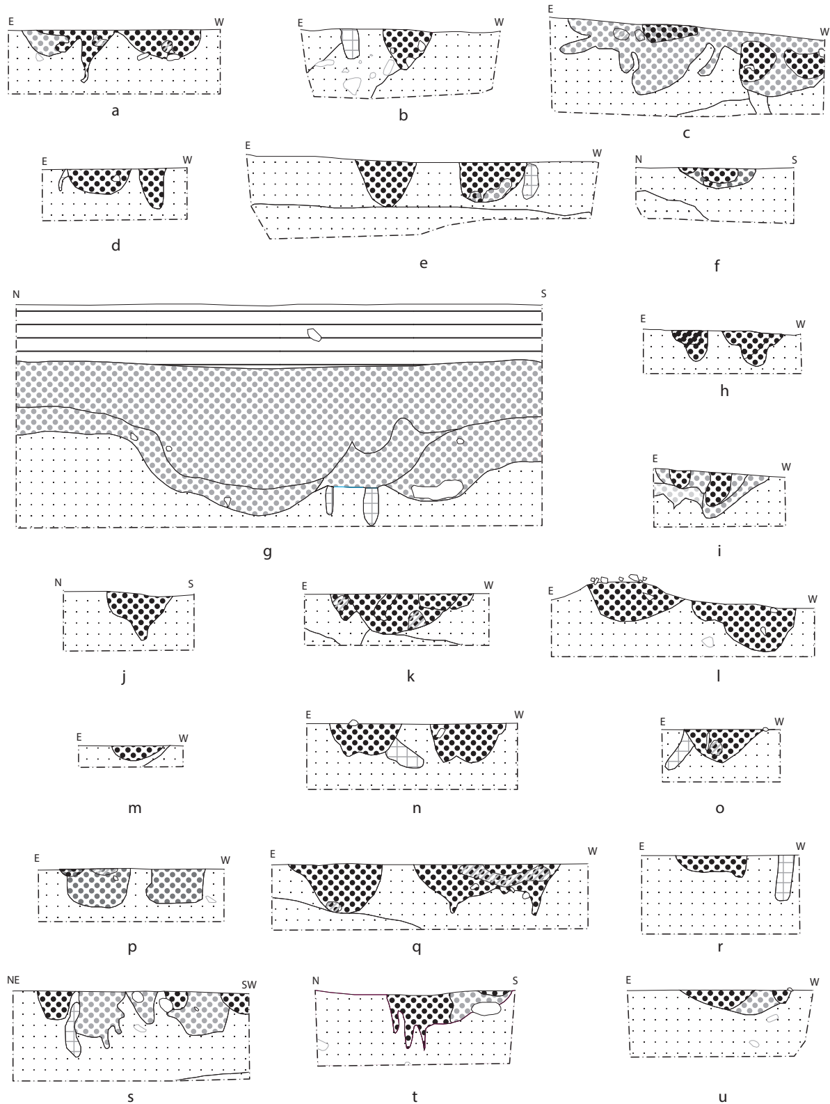
Befundtafel LA22_15 Profile Pfostenlöcher: a: Pr. 83 (Bef. 127); b: Pr. 69 (Bef. 127); c: Pr. 70 (Bef. 82 u. 83); d: Pr. 85 (Bef. 152); e: Pr. 72 (Bef. 166 u. 167); f: Pr. 73 (Bef. 169); g: Pr. 74 (Bef. 170); h: Pr. 75 (Bef. 171 u. 172); i: Pr. 76 (Bef. 173 u. 174); j: Pr. 77 (Bef. 175); k: Pr. 80 (Bef. 134 u. 135); l: Pr. 81 (Bef. 134 u. 135); m: Pr. 92 (Bef. 141); n: Pr. 82 (Bef. 136 u. 138); o: Pr. 86 (Bef. 158); p: Pr. 85 (Bef. 153 u. 154); q: Pr. 87 (Bef. 159 u. 160); r: Pr. 89 (Bef. 163); s: Pr. 90 (Bef. 161 u. 162); t: Pr. 93 (Bef. 144); u: Pr. 94 (Bef. 145). M 1:20.
