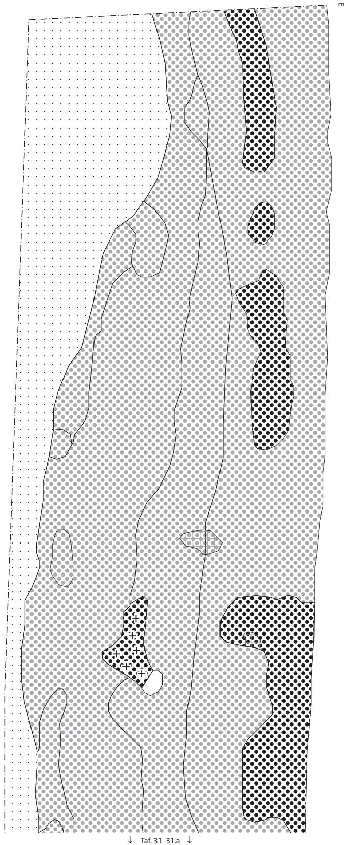
Befundtafel LA31_30 Profile Erdentnahmegrube Pr. 26 (Bef. 4), M 1:20.
