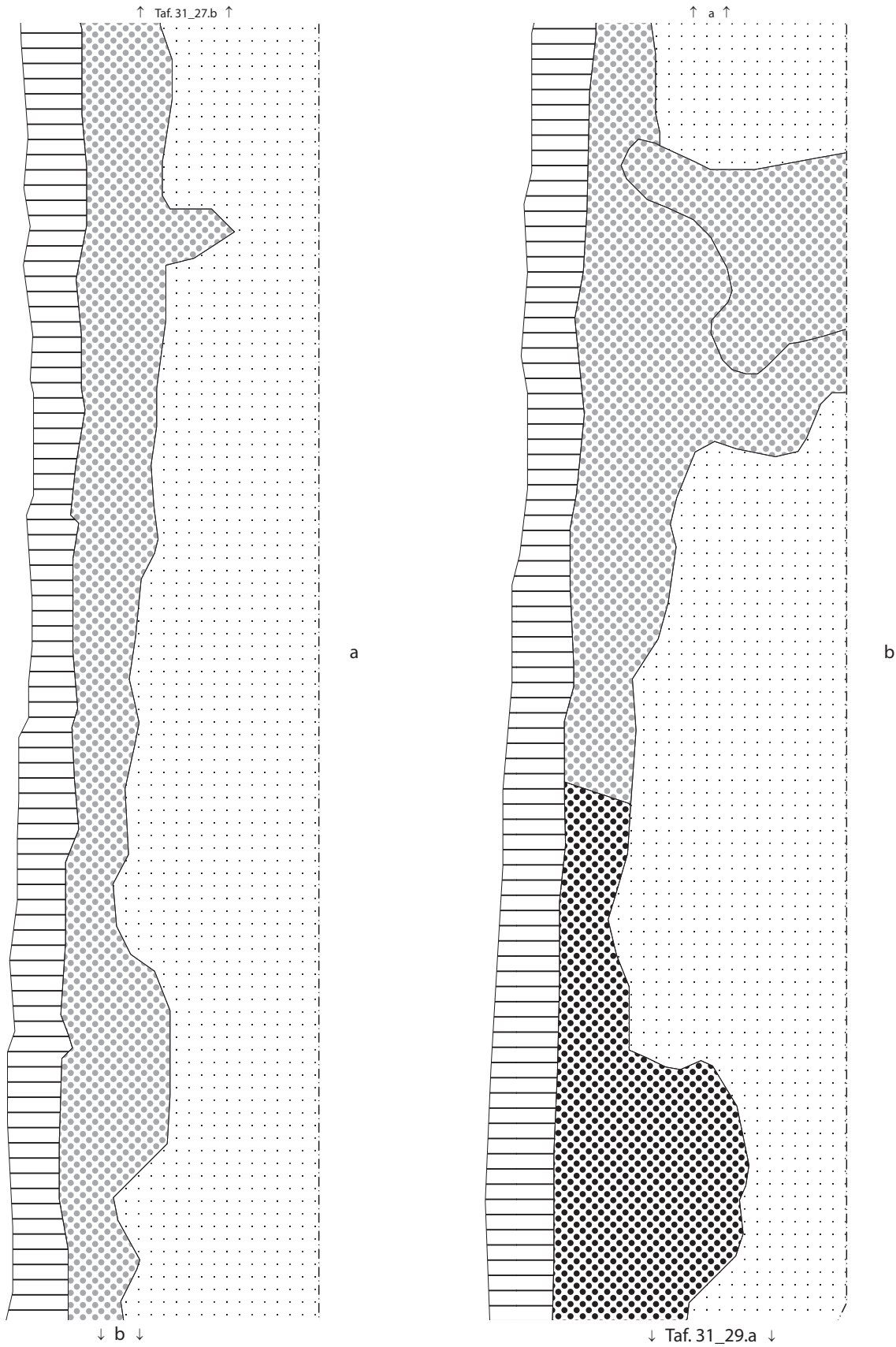
Befundtafel LA31_28 Profile Erdentnahmegrube (Bef. 4) u. Erdgrab (Bef. 29) a u. b : Pr. 31. M 1:20.
