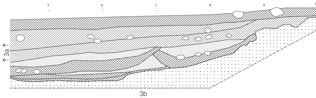
Befundtafel LA1_86 Profil eingehetzte Gruben: 1: Pr_1083; 2: Pr_180; 3: 68. M 1:40.
