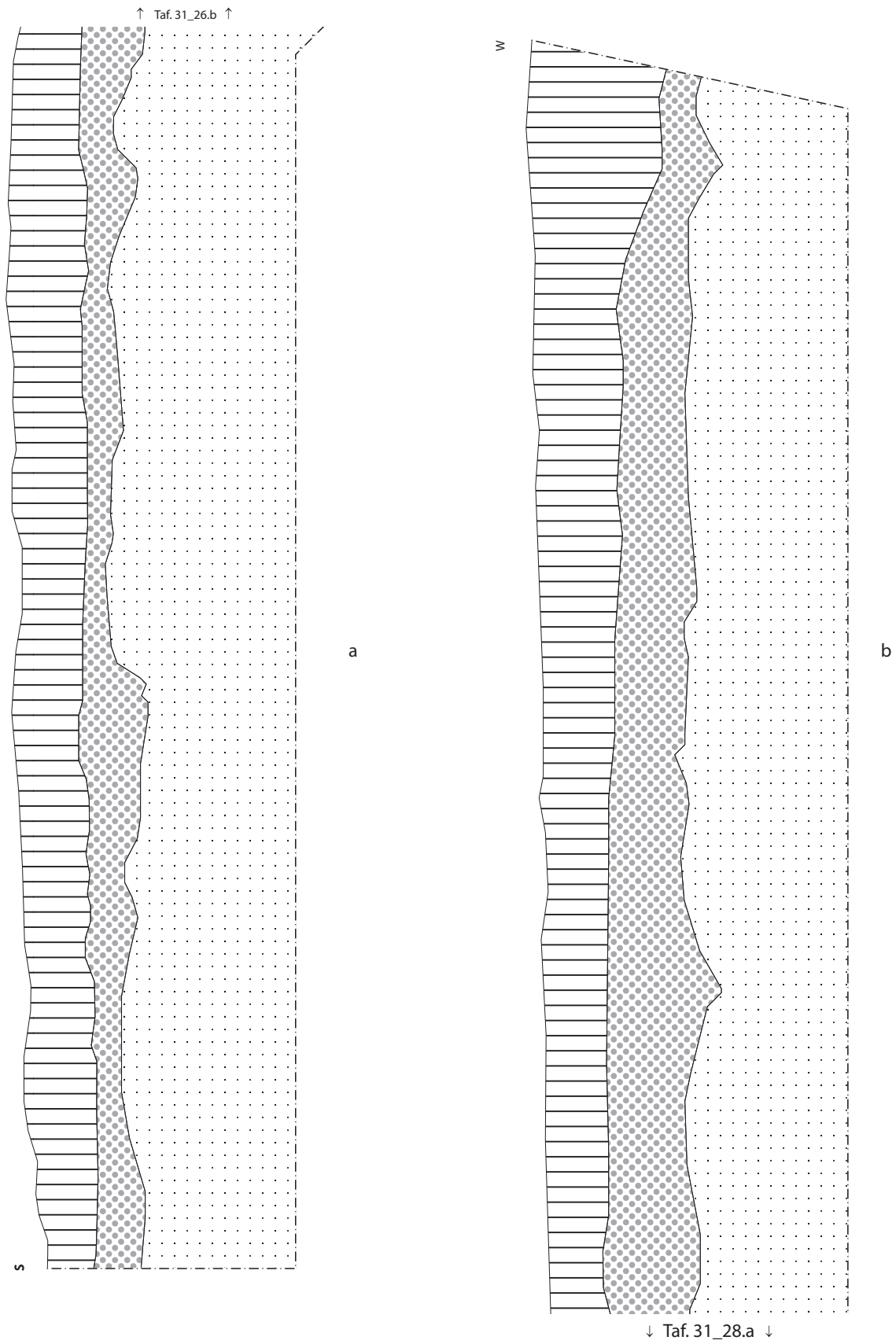
Befundtafel LA31_27 Profile Erdentnahmegrube (Bef. 4) a: Pr. 31; b: Pr. 31. M 1:20.
