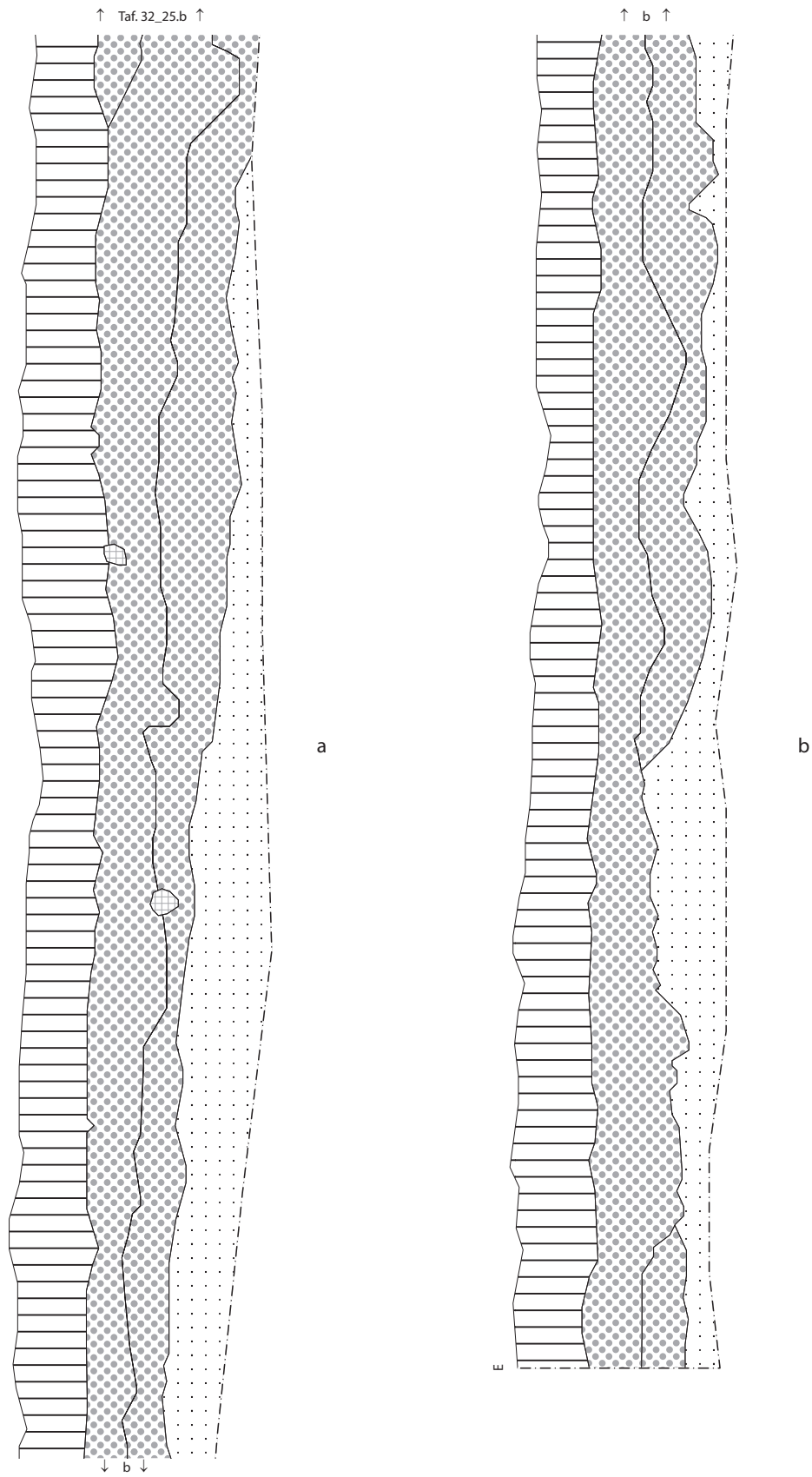
Befundtafel LA32_24 Profil Erdentnahmegrube a u. b: Pr. 24 (Bef. 3). M 1:20.
