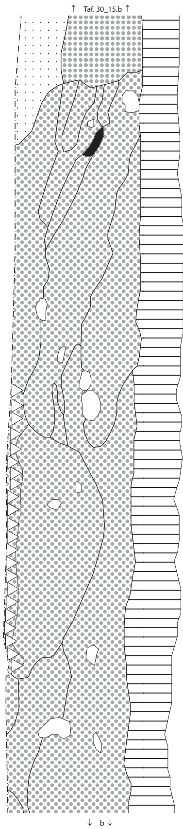
Befundtafel LA30_16 Profile Grabkammer (Bef. 6) Hügelschüttung a u. b: Pr. 7; c: Pr. 21 (Bef. 21_1). M 1:20.
