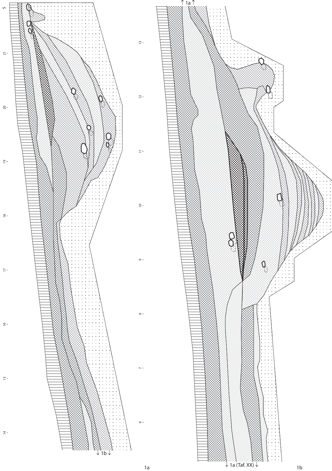
Befundtafel LA1_88 Profil Grabensegment und eingehetzte Grube 1: Pr_1089. M 1:40.
