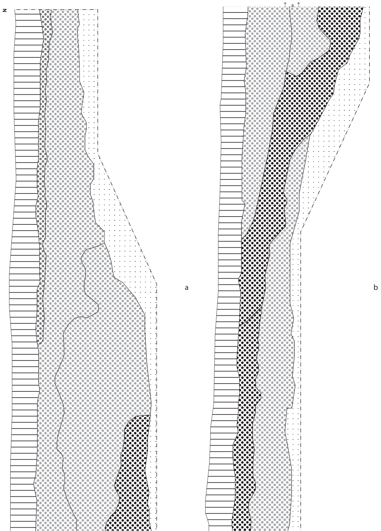
Befundtafel LA31_25 Profile Erdentnahmegrube (Bef. 4) Pr. 29. M 1:20.
