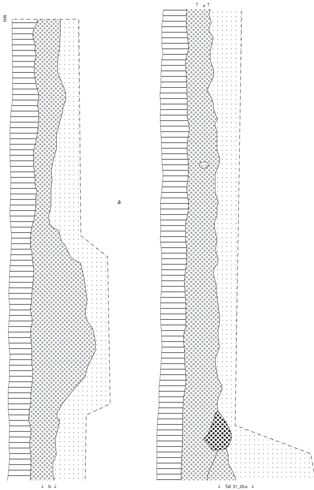
Befundtafel LA31_19 Profile Erdentnahmegrube (Bef. 4) a u. b: Pr. 7. M 1:20.
