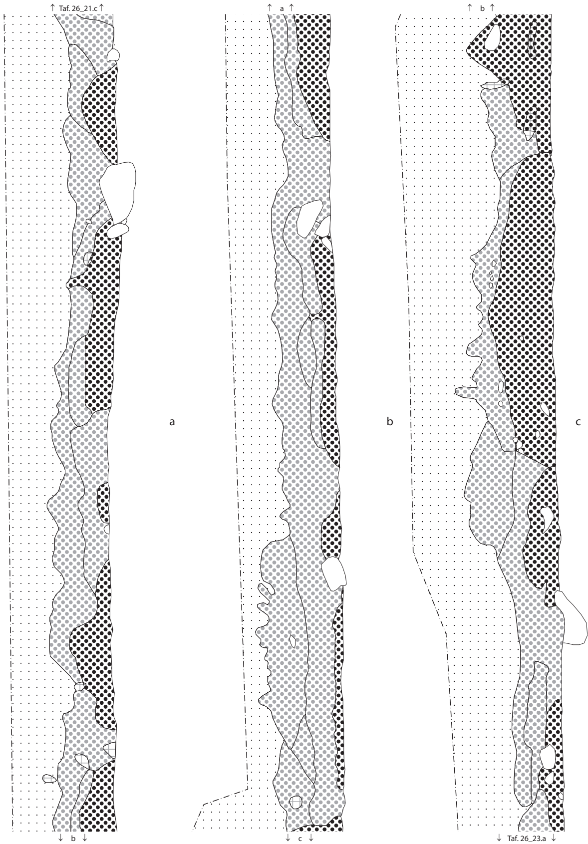
Befundtafel LA26_22 Fundamentgraben und Standgruben a-c: Pr. 7 (Bef. 11; 61; 62; 63; 64; 73; 74; 75; 76; 77; 78; 79). M1:20.
