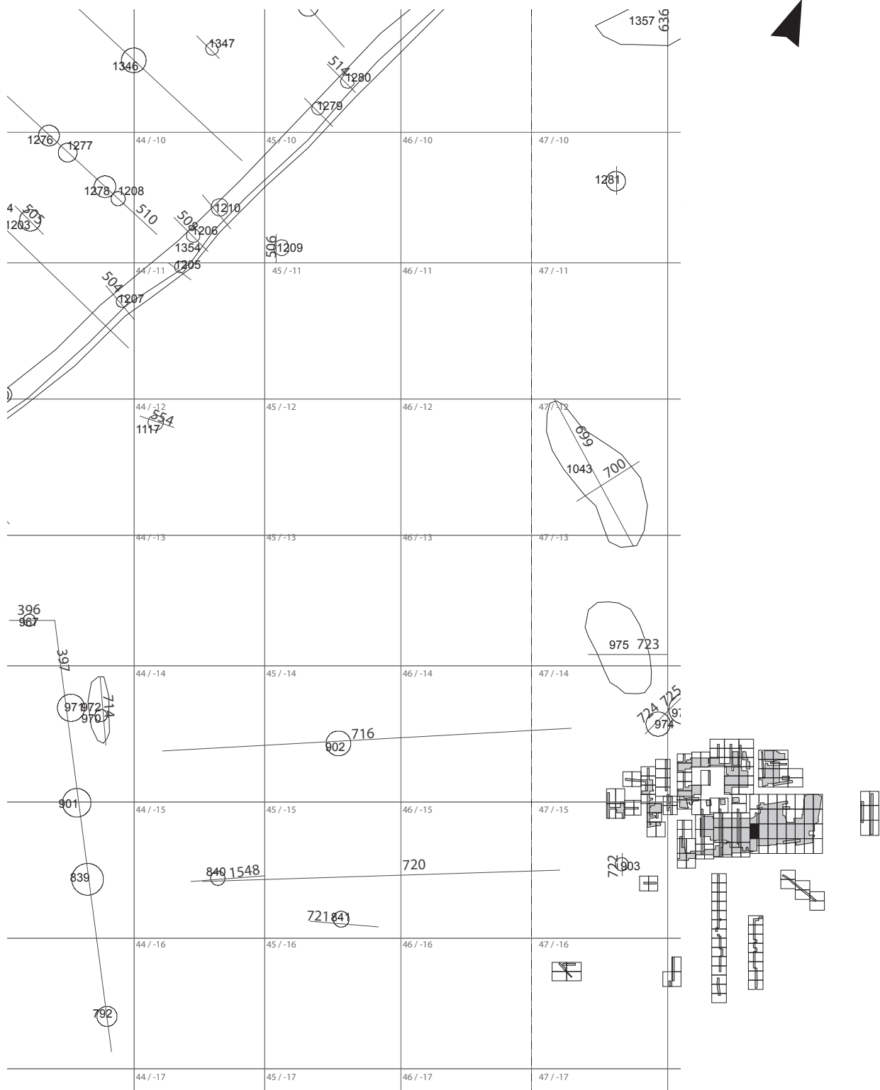
Planum LA 1 - Ausschnitt 80. M 1:125
