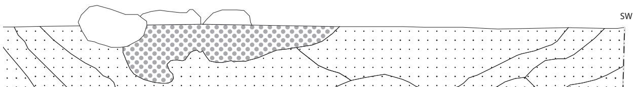
Befundtafel LA28_3 Standgruben a: Pr. 1 (Bef. 1); b: Pr. 2 (Bef. 2); c-d Pr. 4 (Bef. 4); e: Pr. 3 (Bef. 3); f: Pr. 5 (Bef. 5). M 1:20.
