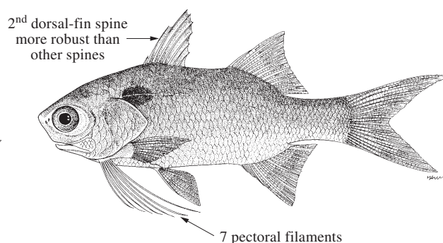
Fig. 68 Polydactylus mullani
