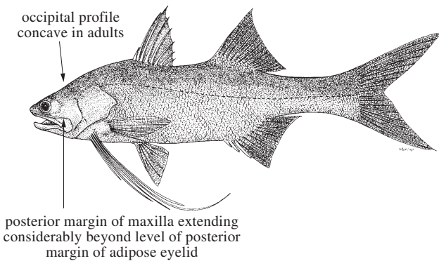
Fig. 72 Polydactylus macrochir
