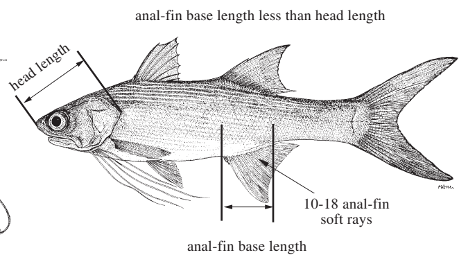
Fig. 15 Polydactylus bifurcus
