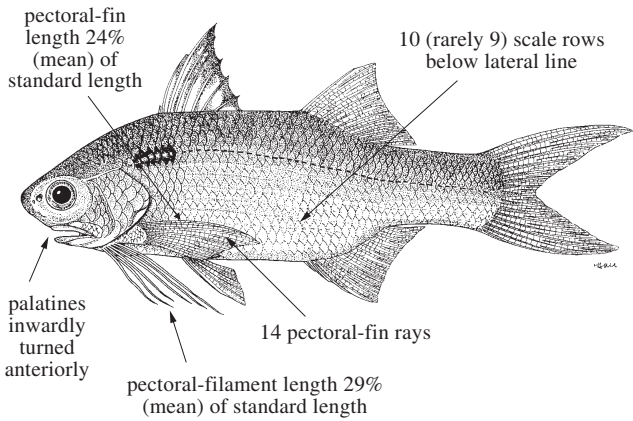
Fig. 70 Polydactylus malagasyensis
