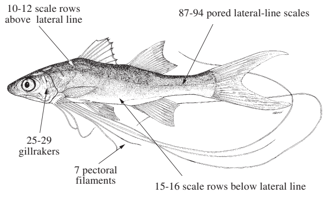
Fig. 77 Polydactylus macrophthalmus
