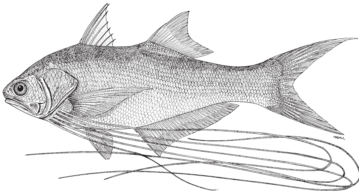
Fig. 65 Pentanemus quinquarius
