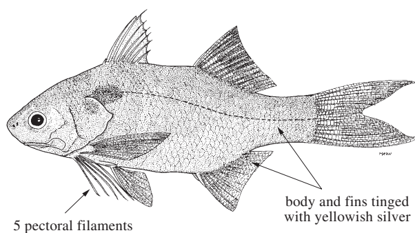
Fig. 67 Polydactylus microstomus
