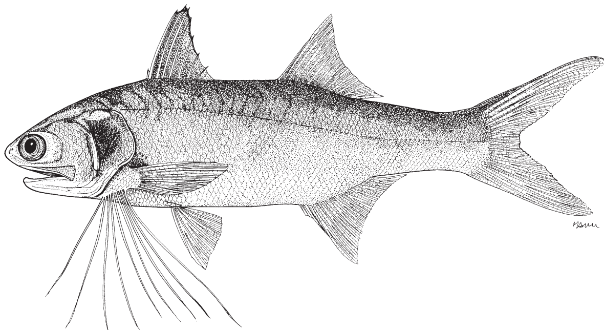
Fig. 112 Polydactylus opercularis
