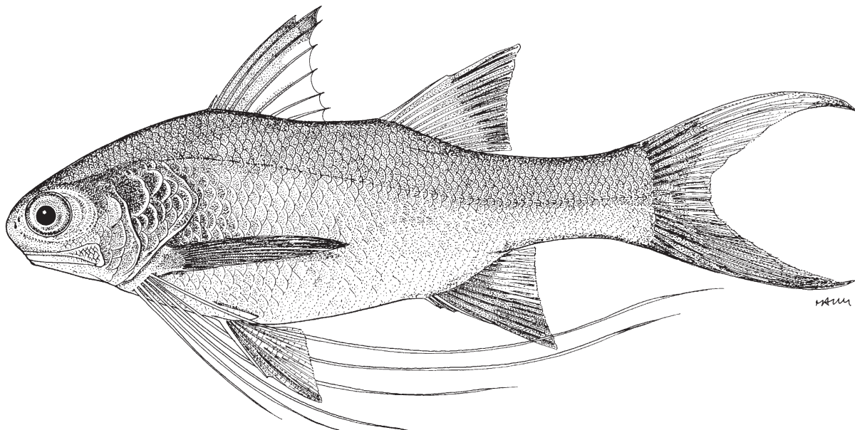
Fig. 91 Polydactylus longipes
