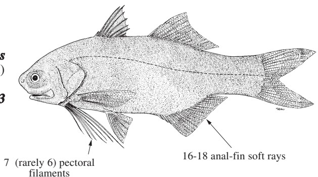
Fig. 78 Polydactylus multiradiatus
