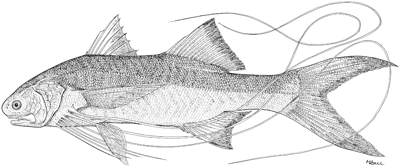
Fig. 136 Polynemus aquilonaris
