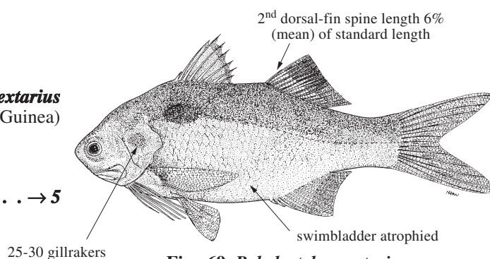
Fig. 69 Polydactylus sextarius
