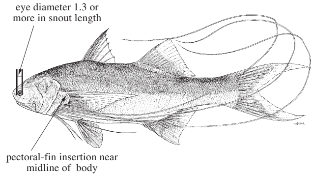
Fig. 11 Polynemus paradiseus
