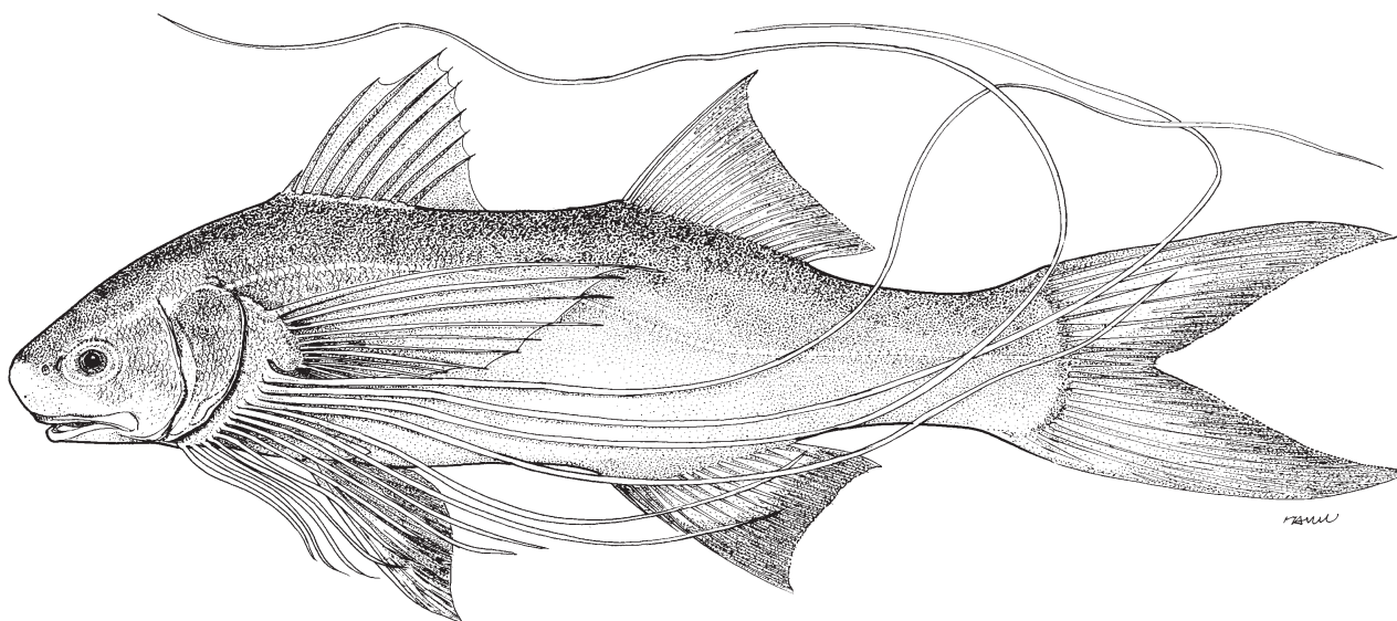
Fig. 148 Polynemus multifilis
