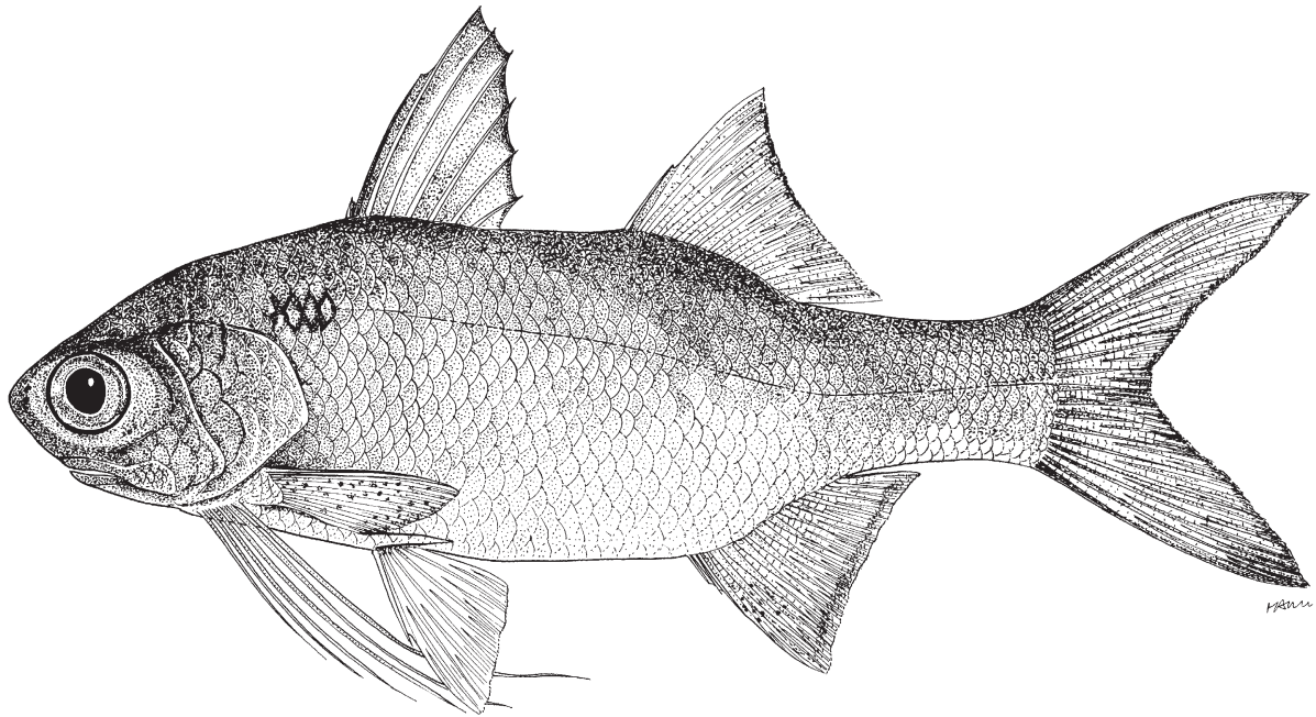
Fig. 114 Polydactylus persicus
