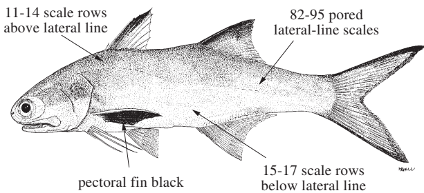
Fig. 33 Eleutheronema rhadinum
