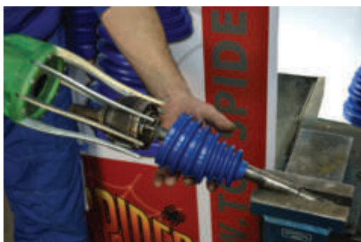
6. PULL OUT THE TOOL FROM THE CV BOOT / Izvući aparat za montažu iz manžetne
