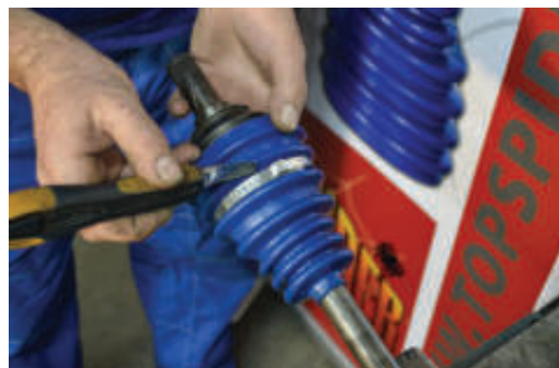
8. CUT THE CV BOOT TO APPROPRIATE DIMENSIONS / Iseći manžetnu na odgovarajuću dimenziju
