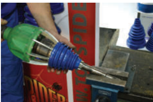
5. DROP THE AIR FROM THE TOOL / Ispustiti vazduh iz aparata za montažu
