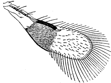
Fig. 3. — Casca luzonica Malen. Ala anteriore della femmina, ingr. 116 diam.
