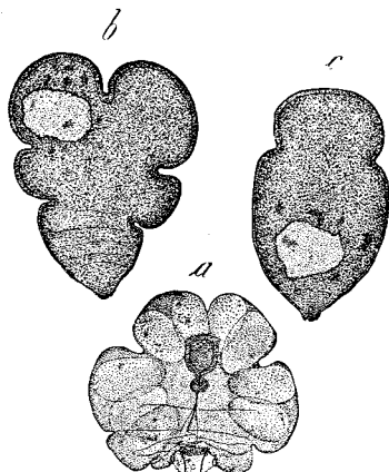
Fig. 6. — Schizaspis lobata Cockll. e Rob. a) Femmina ovigera sana, vista dal ventre; b) Femmina uccisa dalla Casca luzonica Malen., vista dal dorso. c) Ninfa uccisa dalla Casca luzonica Malen., vista dal dorso. Ingr. 43 diam.
