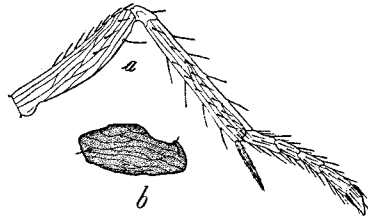
Fig. 5. — Casca luzonica Malen. Femmina. a) Femore, tibia e tarso della zampa mediana; b) anca posteriore. Ingr. 182 diam.
