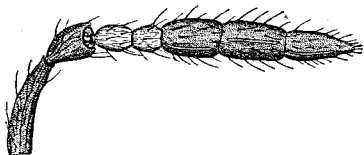
Fig. 1. — Casca luzonica Malen. Antenna della femmina, ingr. 182 diam.
