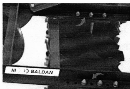
Regulagens para aumentar ou diminuir o ângulo de corte dos discos. Adjustments to increase or decrease the cutting angle of the discs. Ajustes para aumentar o disminuir el ángulo de corte de los discos.
