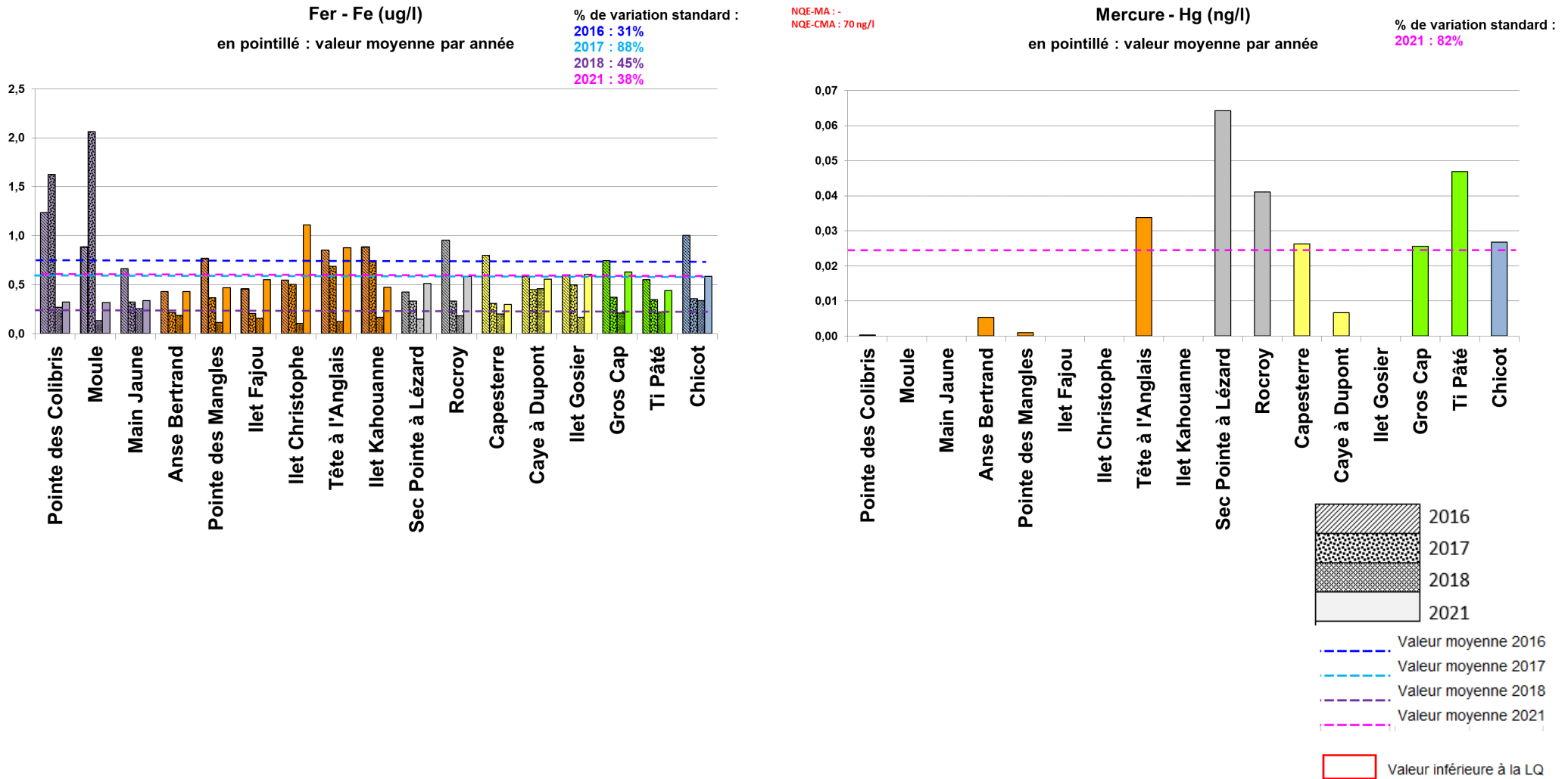
Figure 8 - Concentrations DGT moyennes des contaminants métalliques Fe et Hg mesurées sur les 17 stations DCE de Guadeloupe lors des campagnes de 2016, 2017, 2018 et 2021
