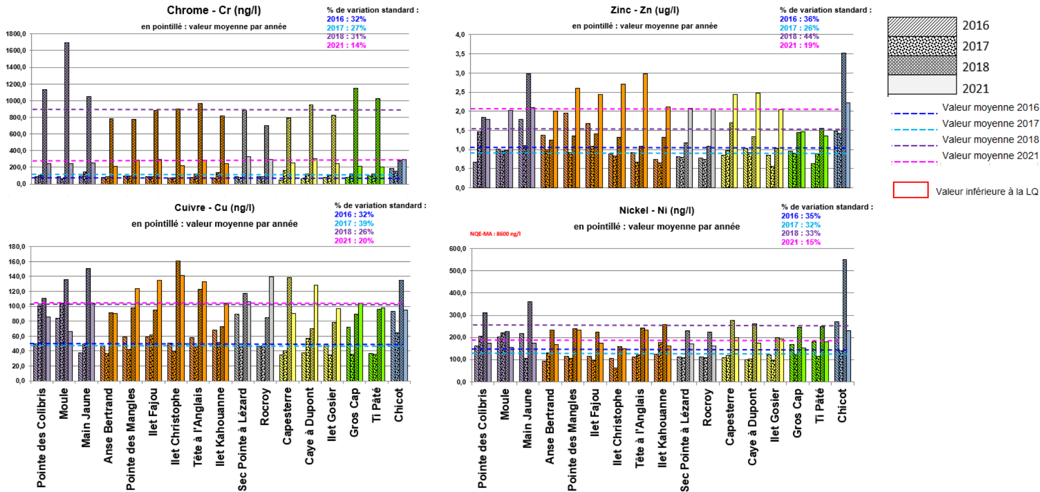
Figure 7 - Concentrations DGT moyennes des contaminants métalliques Cr, Cu, Zn et Ni mesurées sur les 17 stations DCE de Guadeloupe lors des campagnes de 2016, 2017, 2018 et 2021
