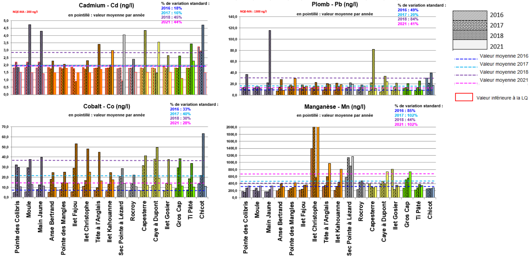
Figure 6 - Concentrations DGT moyennes des contaminants métalliques Cd, Co, Pb et Mn mesurées sur les 17 stations DCE de Guadeloupe lors des campagnes de 2016, 2017, 2018 et 2021
