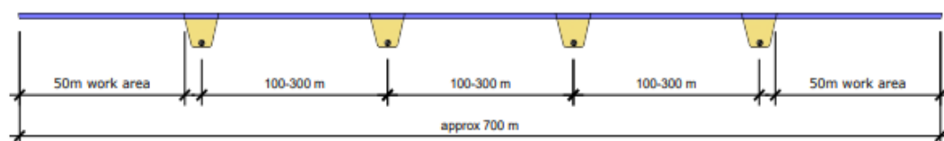
Figur 13: Exempel på avstånd som kan komma att krävs vid förläggning av växelströmskablar (HVAC) till havs.
