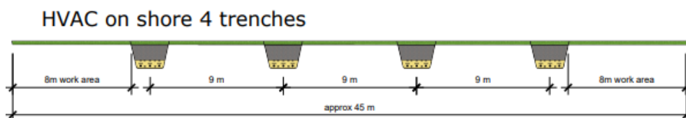
Figur 9: Ytor som generellt krävs vid användning av växelströmskablar (HVAC).
