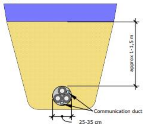
Figur 12: Exempelskiss på schaktprofil för sjökabel av växelströmstyp (HVAC) till havs.
