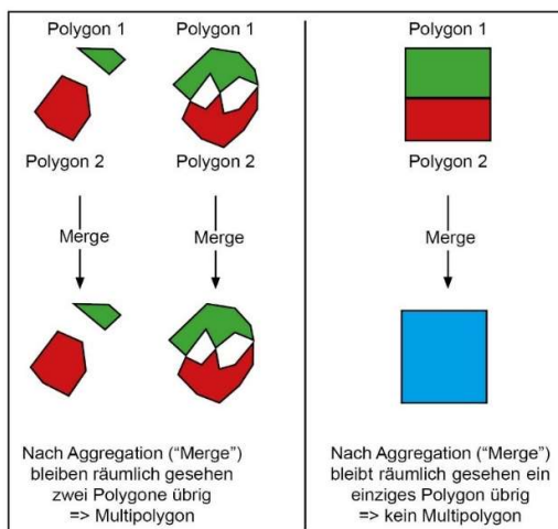
Abbildung 2: Definition Multipolygon
