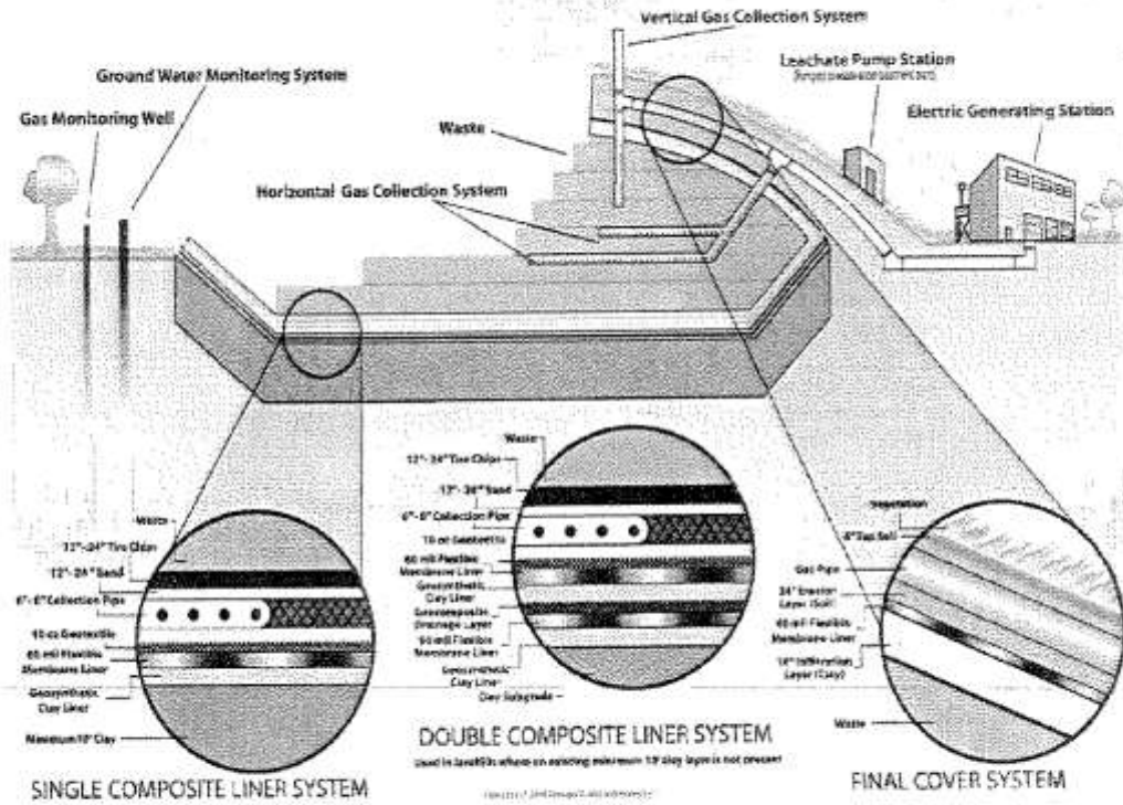
Figure 9 Μια άλλη κατασκευή ΧΥΤΑ. Παρατηρείστε την διπλή κατασκευή για ενίσχυση στον πυθμένα.
