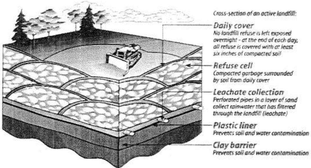
Figure 11 Τομή ενός ΧΥΤΑ σε λειτουργία
