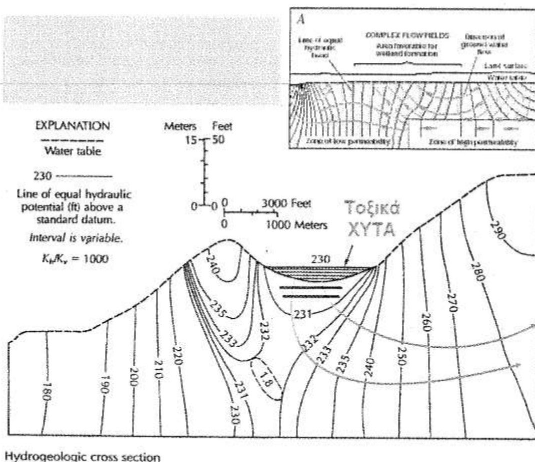
Figure 3 Υδρογεωλογικό μοντέλο που θα έπρεπε να υπάρχει
