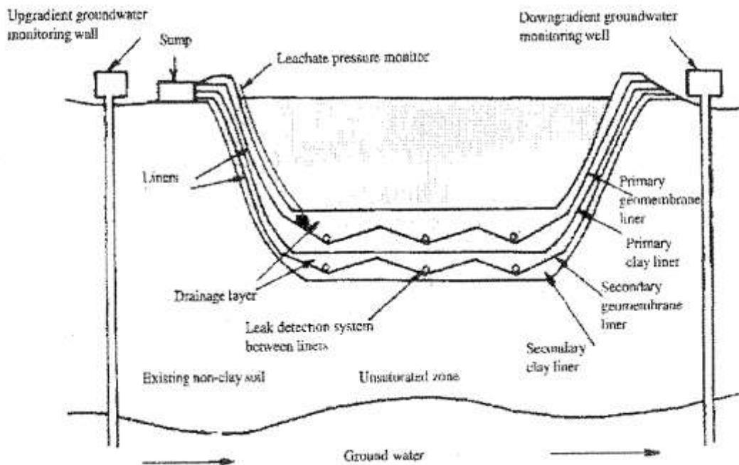
Figure 10 Κατασκευή χιτώνια ΧΥΤΑ. Χρήση ειδικών ανιχνευτών.
