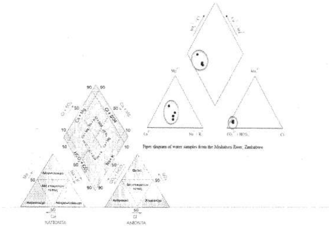
Figure 15 Κύριοι υδροχημικοί τύποι στο διάγραμμα Piper
