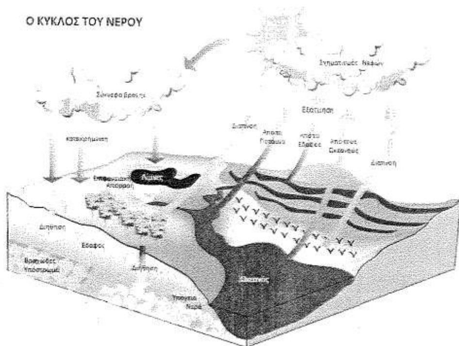
Figure 7 Ο Κύκλος του Νερού
