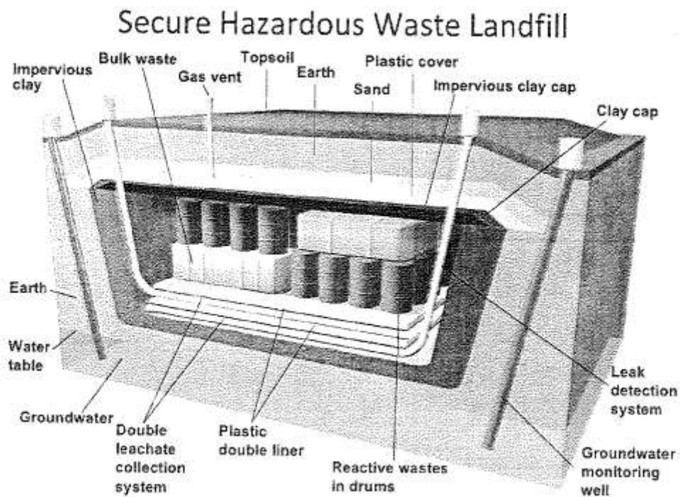
Figure 8 ΧΥΤΑ για επικίνδυνα απόβλητα
