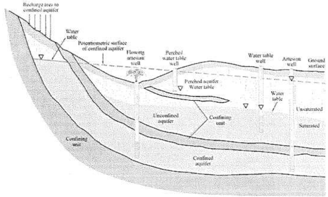
Figure 14 Σχηματισμός πηγαδιών από υπέργεια και υπόγεια ύδατα
