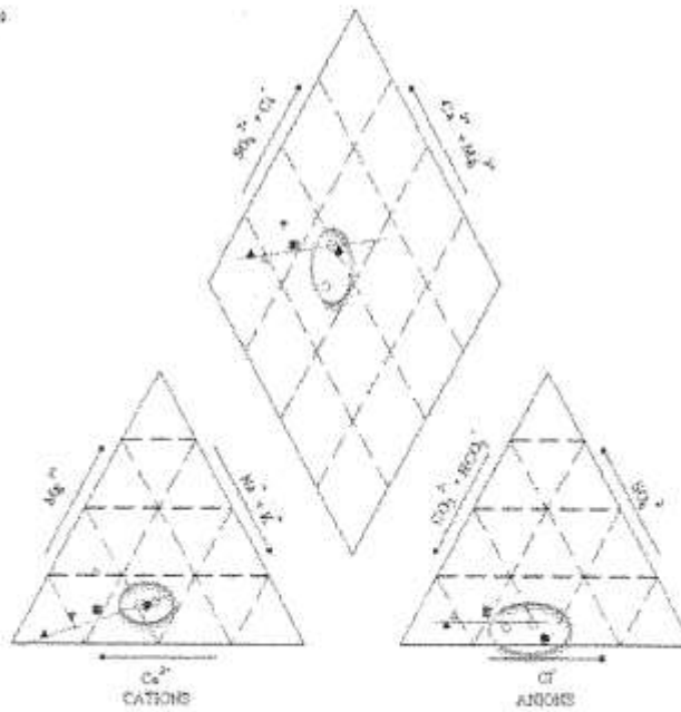
Figure 16 Διαγράμματα Piper στα δεδομένα μελέτης IGME (οι ευθείες προστέθηκαν από εμένα)
