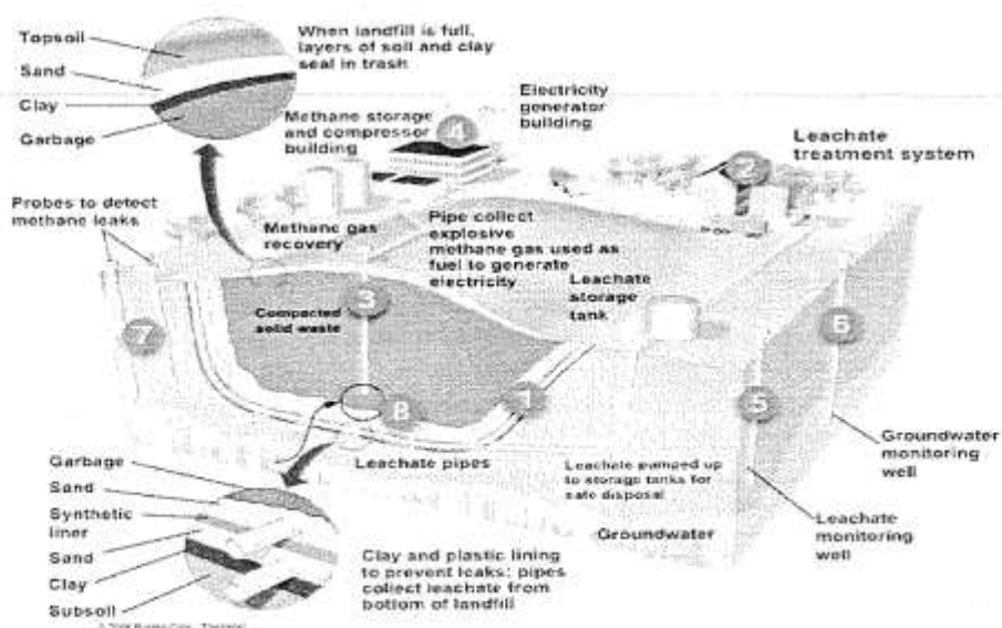
Figure 2 Εννοιολογική κατασκευή ενός ΧΥΤΑ
