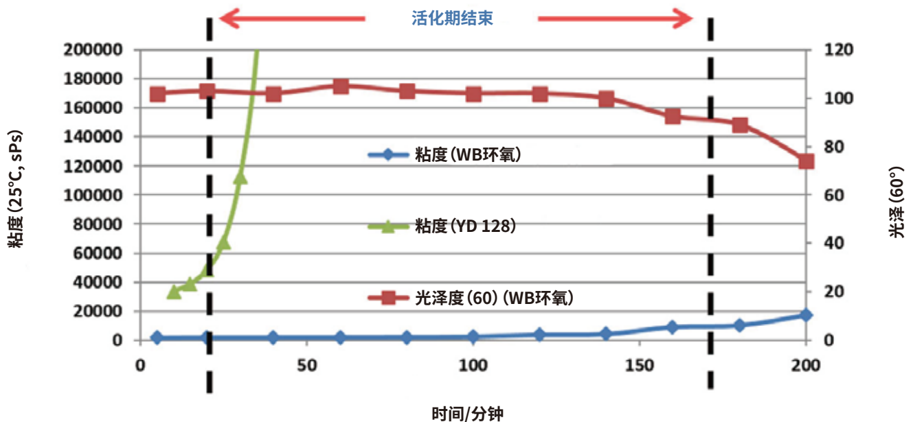
图5 图中显示了使用相同固化剂固化的水性1型环氧乳液 (wb环氧) 和液体环氧树脂 (yd 128) 的粘度上升曲线图。
