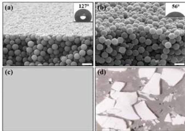
图4 ❖ 冲洗后漆膜的SEM图像和照片: a) 由Janus颗粒形成的漆膜; b) 具疏水颗粒的漆膜; c) 冲洗后添加Janus颗粒的漆膜照片; d) 冲洗后添加均匀颗粒的漆膜照片。比例尺均为2 μm。
