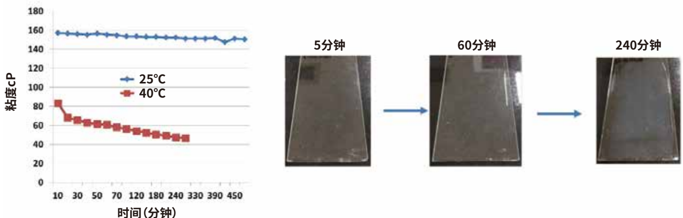
图8 ❖ 基础体系（树脂和固化剂）的粘度状态和成膜行为。
