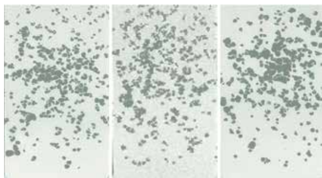
图6 ❖ PC-WPU 样板的低温抗石击结果。
