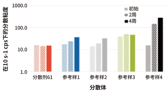
图6 工业碳黑1分散体的高温稳定性。黑色：15%的PBK-，100% SOP的分散剂用量。
