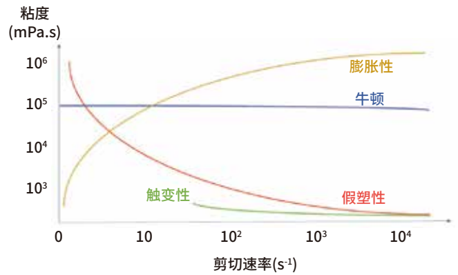
图1 粘度与剪切速率：牛顿、膨胀性、假塑性和触变流体。
