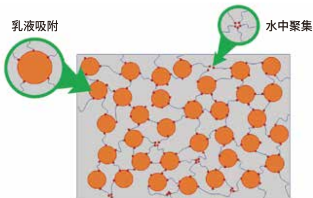
图4 ❖ 缔合型增稠剂的工作原理。
