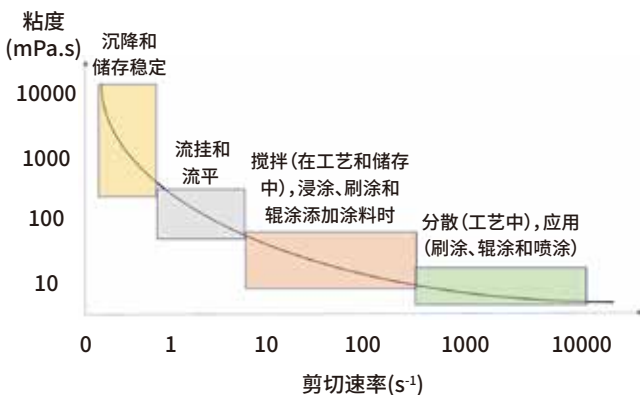
图3 ❖ 普通涂料应用的粘度和剪切速率范围。
