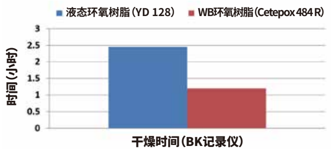
图6 用同一固化剂固化的水性1型环氧乳液 (wb环氧) 和液体环氧树脂 (yd 128) 的干燥时间曲线图。
