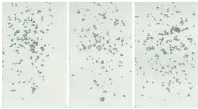
图4 ❖ PET-WPU-2 样板的低温抗石击结果。
