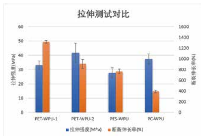
图7 ❖ 不同 WPU 干膜的拉伸测试对比。
