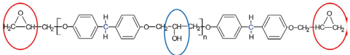
图2 ❖ 标准环氧树脂的反应位置。
