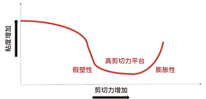
图2 涂料的粘度曲线。
