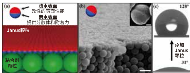
图3 ❖ a) 涂层结构示意图; b) 涂层结构横截面图的SEM图像。比例尺为2 μm。插图显示了典型的Janus颗粒的非对称形态。比例尺为100nm; c) 加入Janus颗粒前后涂层表面的接触角。
