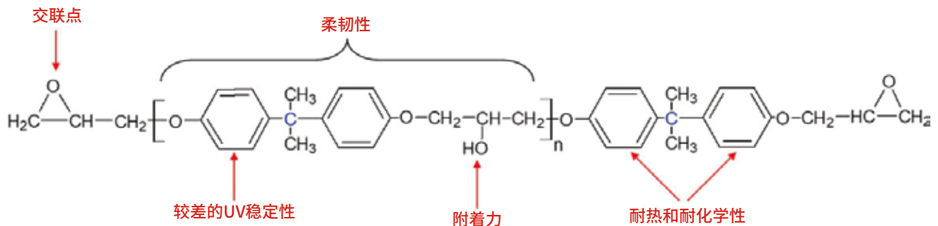
图1 ❖ 双酚A二缩水甘油醚(BADGE)环氧树脂的化学结构。
