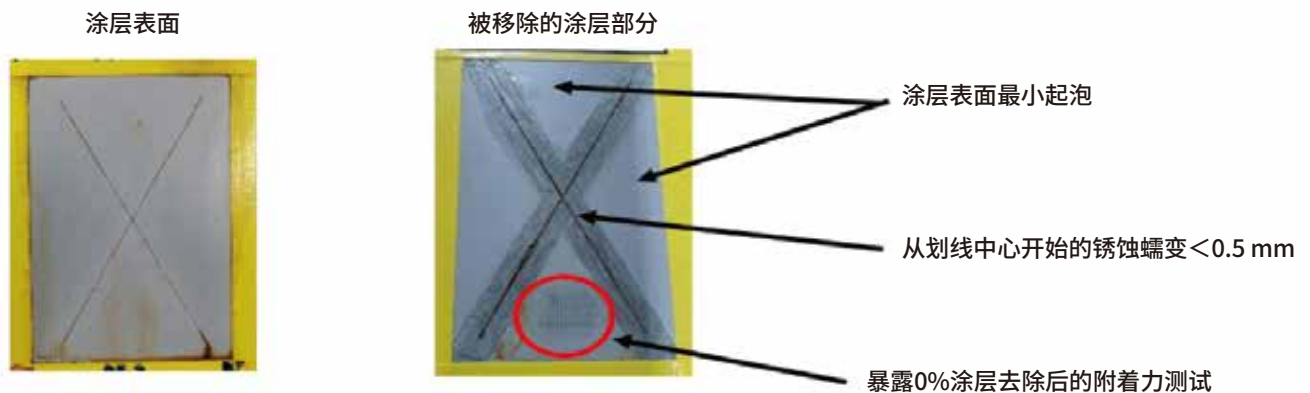
图 10 ❖ 2000小时盐雾暴露后涂层样板的外观 (ASTM B117)。
