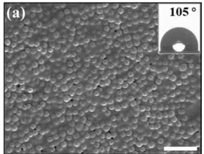
图5 ✦ 添加Janus颗粒的市售底漆粘合剂形成的涂层的SEM图像。比例尺为2 μm。
