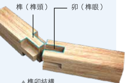
▲榫卯結構
