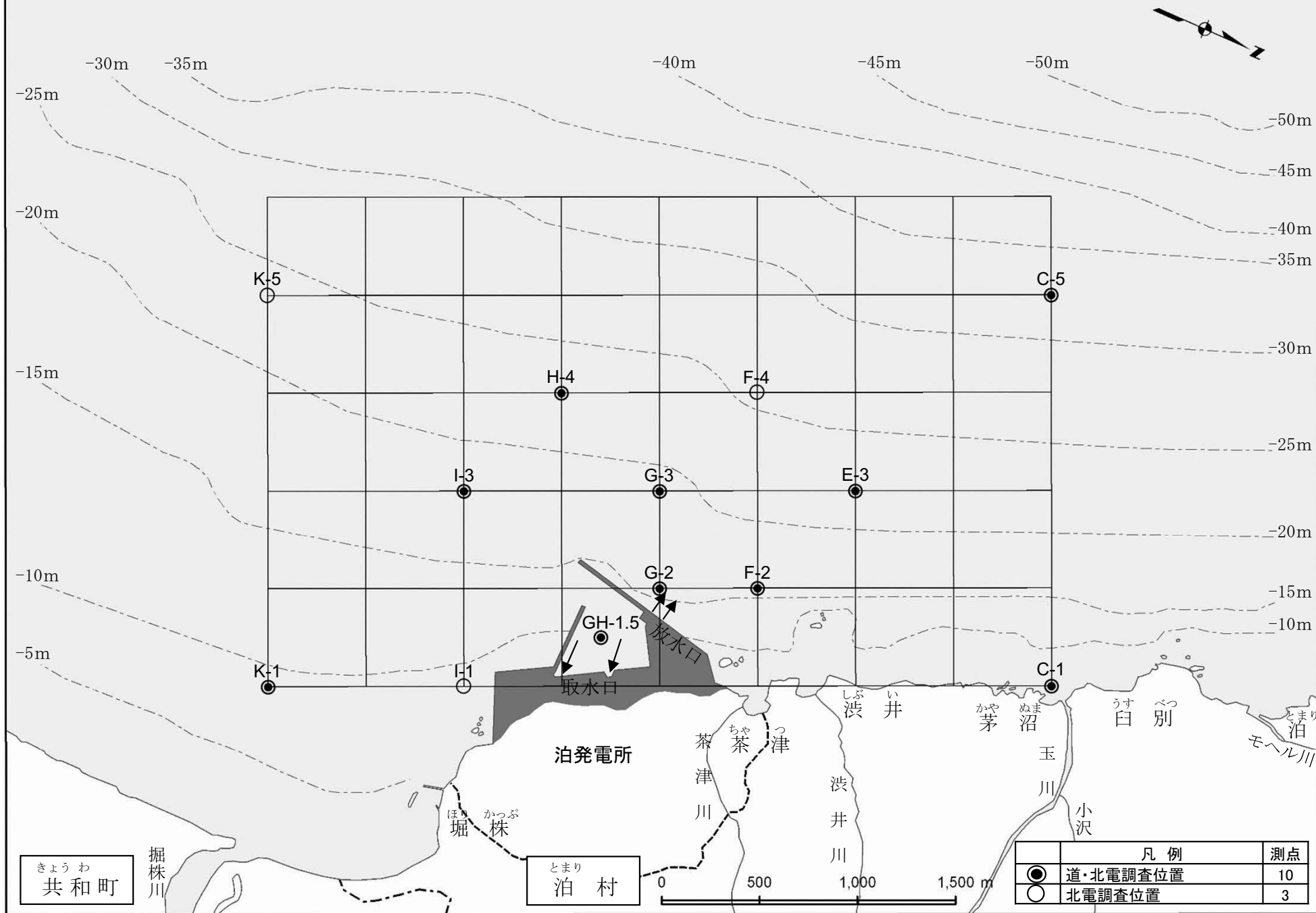
付図-5 底質調査位置
