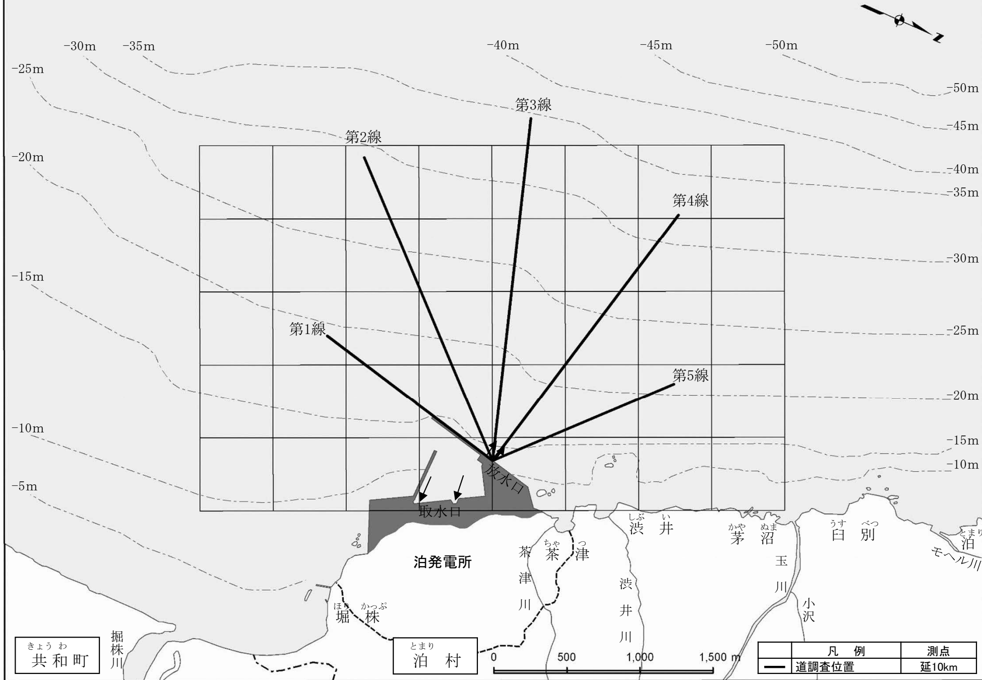
付図-2 水温調査位置(曳航測定)
