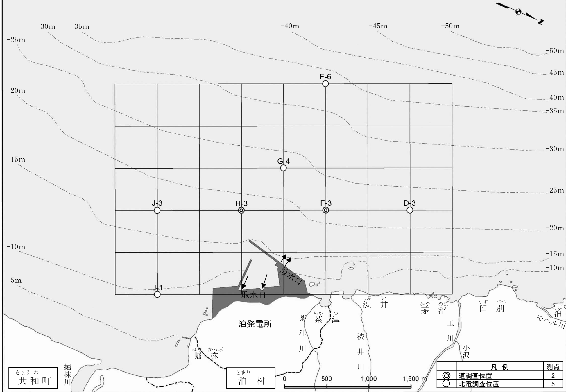
付図-3 流況(流向・流速)調査位置
