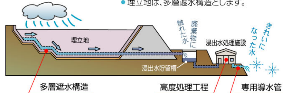
※工事中の濁水は濁水処理プラントを設置し、浄化処理後に放流します。
