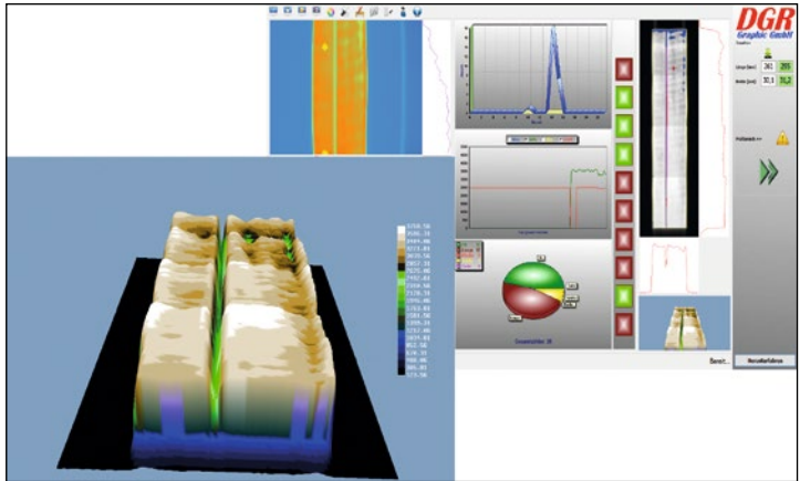
Visualisierung und komplette Inspektion des Leimauftrags mit dem mikrobiologischen Leimkontrollsystem DGR GC.
