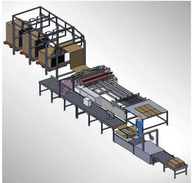
Die Ware wird im Verpackungsprozess gescannt, um die Größe für den individuellen Versandkarton zu berechnen.
