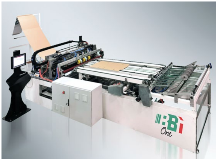
BBI 500 – das Inlinesystem zur individuellen Herstellung von Versandkartons.
