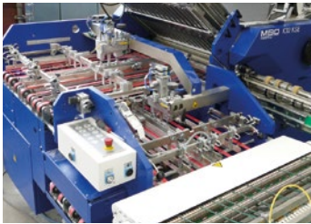
Steubers Beratungskompetenz bei der Kombifalzmaschine MBO K32 KSE, dem Hugo-Beck-Einschweißautomaten oder dem Schnellschneider baumannperfecta 80 liegt im Detail. Jan Gesterkamp vom Steuber-Vertrieb kennt alle Feinheiten.
