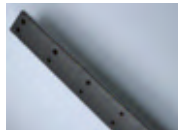
Die 12 (!) mm Ultraflach-Saugdüse arbeitet mit 8 Sauglöchern und deckt 22 x 4 cm Saugfläche in einem Zug ab.
