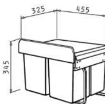
2-fach Trennung Abmessungen: 455 x 345 x 325 mm
