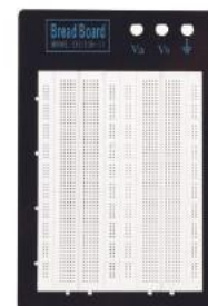
Protoboard 1360 Posições • Protoboard 1360 posições • Com terminais • Connfly 031930
