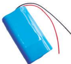
3,7V 1S2P • 38x20x68mm • c/ placa PCM MOD 1 036217 - 4400mAh 036218 - 5200mAh 036329 - 6000mAh
