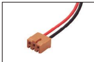
JAEILG-3P • Conector fêmea para uso geral e Telefonia • Rabicho: 15cm 030008
