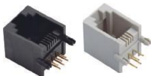
Jack Modular • 4P4C PCI 003144 - 180° PT 003142 - 90°CZ
