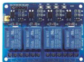
Placa MOD 4R • Modulo com 4 reles p/ robótica 036102
