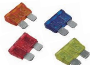
Fusível Automotivo • 32V • Va - Lamina • Emb: 10 pçs 036205 - 15A 036203 - 7,5A 036206 - 20A 036204 - 10A 036207 - 40A
