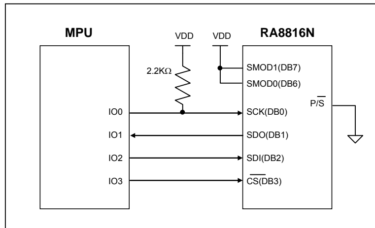
圖 6-5 : 4 線式 (B-Type) 的 MPU 介面圖
