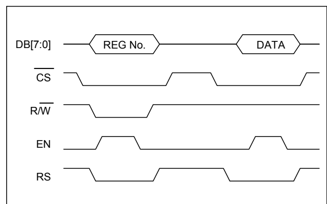
圖 6-9：以 6800 8-bit 對暫存器讀取的時序圖
