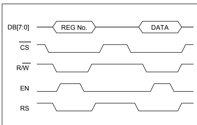
圖 6-8：以 6800 8-bit 對暫存器寫入的時序圖
