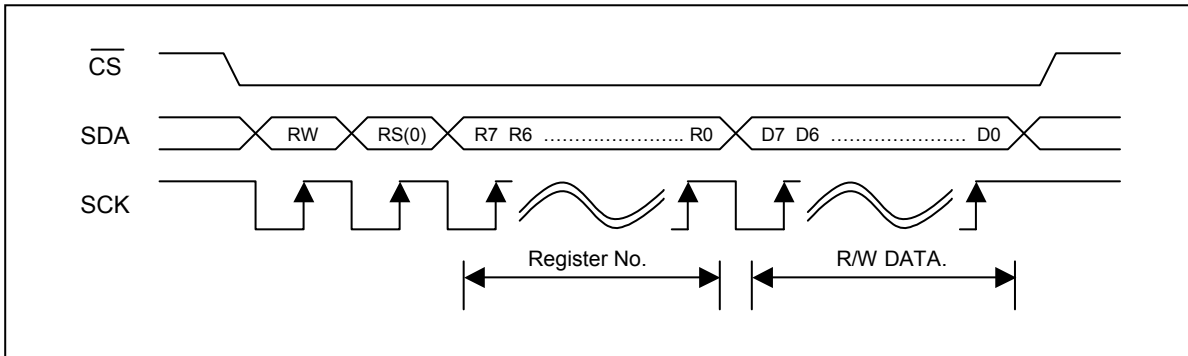
圖 6-10 : 3 線串列介面對暫存器讀寫的時序圖
