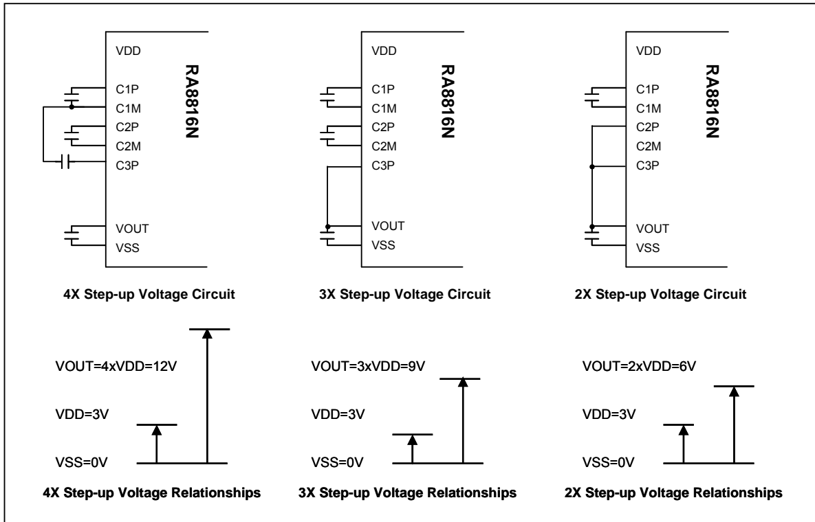
圖 6-22：步階升壓應用電路
