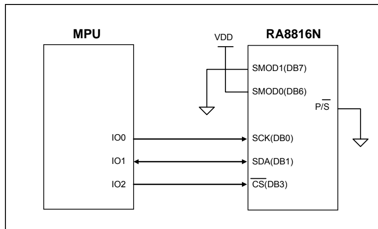
圖 6-3：3 線式的 MPU 介面圖
