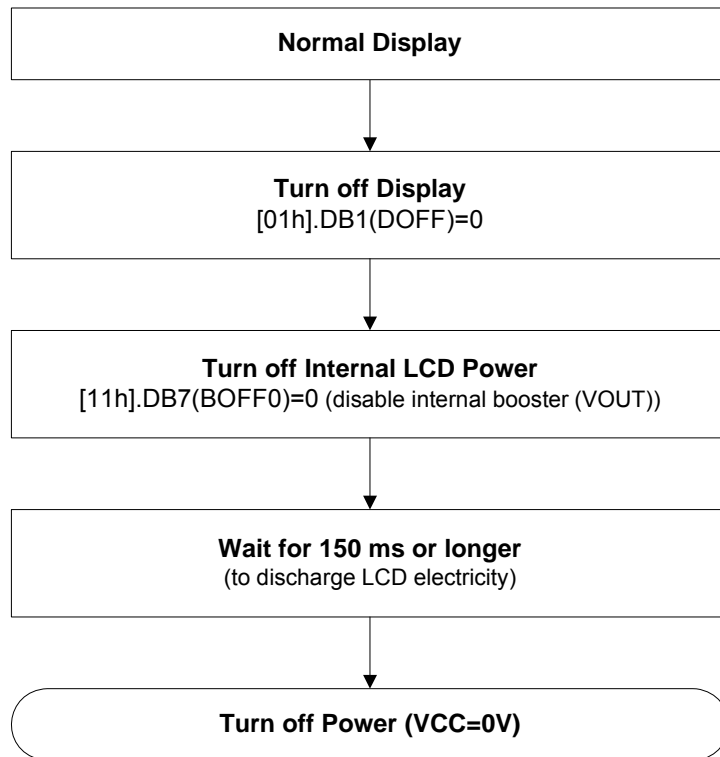
圖 6-35 : 電源關閉順序
