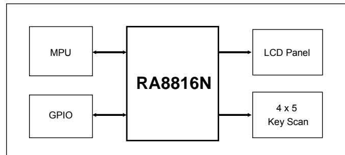
圖 3-1 : System Block
