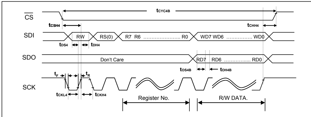
圖 9-5 : 4-Wire (B Type) 時序
