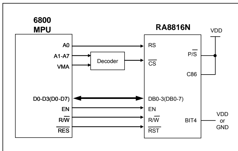
圖 6-2 : 6800 (4/8-Bit) MPU Interface
