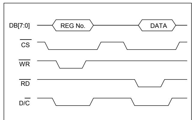
圖 6-7：以 8080 8-bit 對暫存器讀取的時序圖
