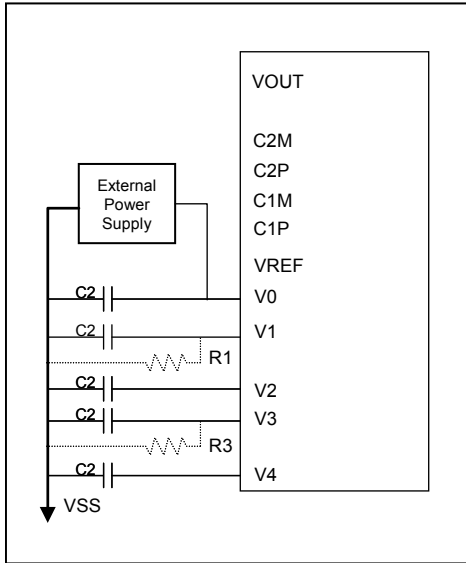
圖 6-27：使用內部電壓隨耦器
