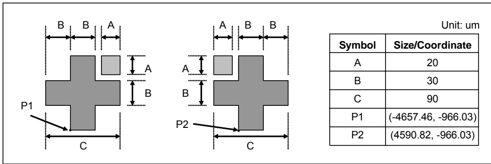
圖 8-2：定位點尺寸
