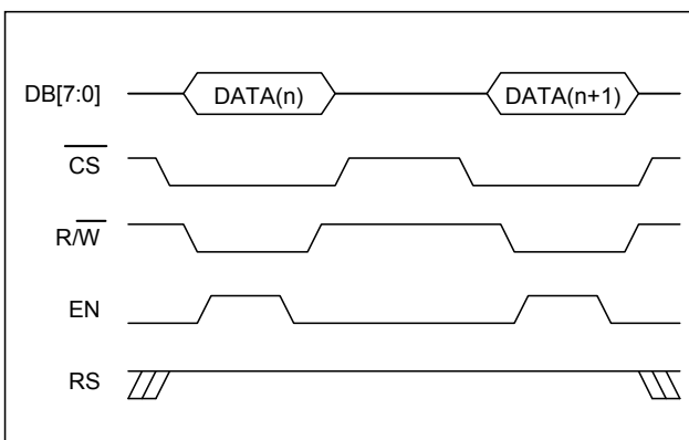
圖 6-15：以 6800 8-bit 對記憶體寫入的時序圖
