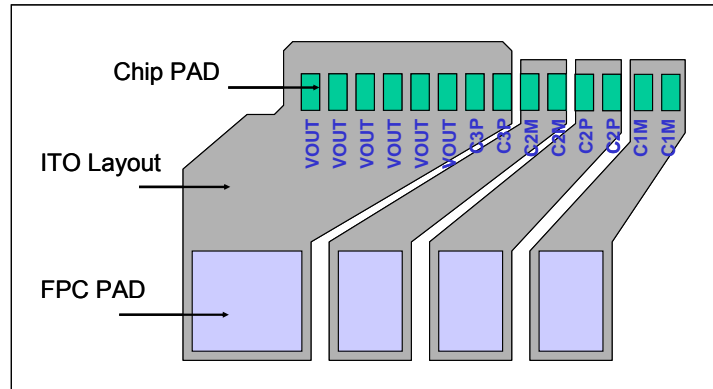
圖 A-7：ITO 走線範例 - VOUT
