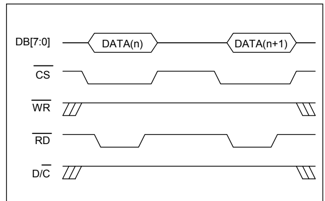
圖 6-14：以 8080 8-bit 對記憶體讀取的時序圖
