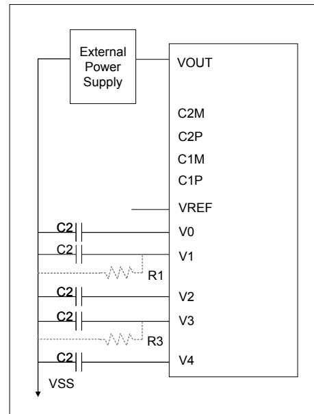
圖 6-24：使用外部 VOUT 電源電路
