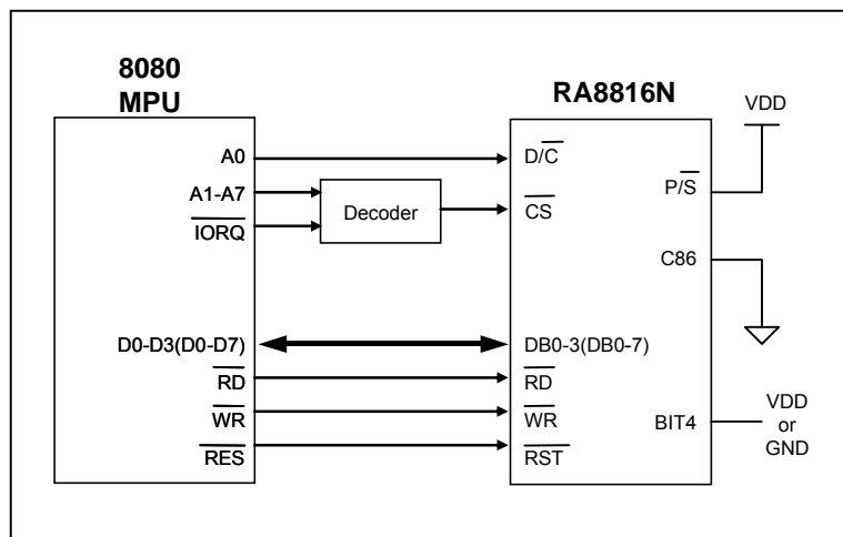
圖 6-1 : 8080 (4/8-Bit) MPU Interface
