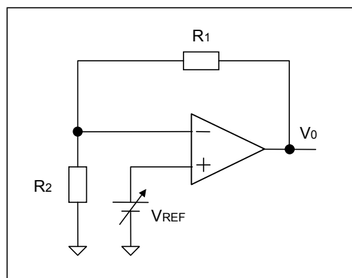
圖 6-25：電壓隨耦器
