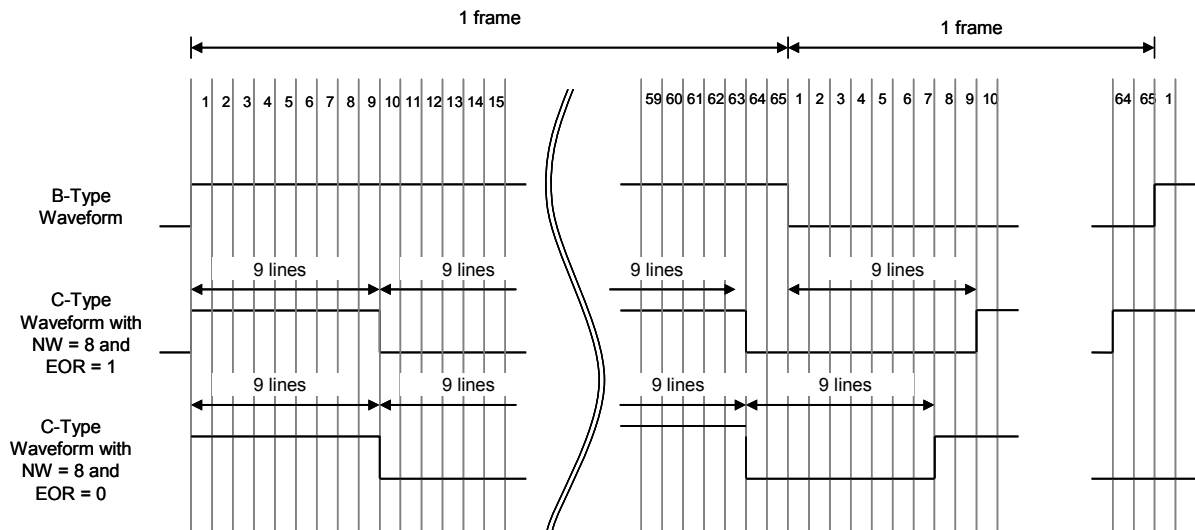
圖 6-20 : N-Line 反轉波型圖
