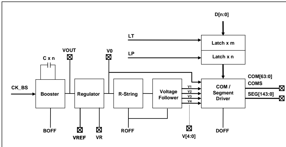
圖 6-21 : LCD 驅動器與電壓供應電路方塊圖
