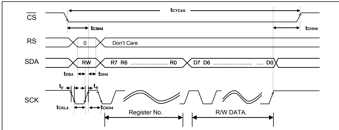
圖 9-4 : 4-Wire (A-Type) 時序
