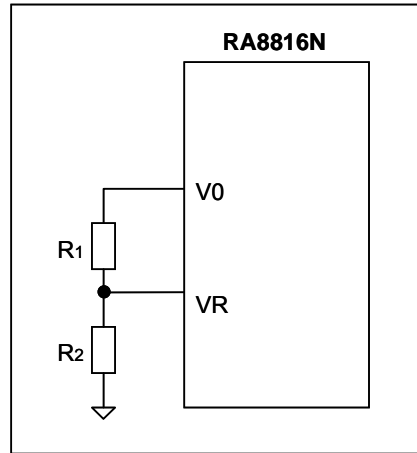
圖 6-26：使用外部分壓電阻
