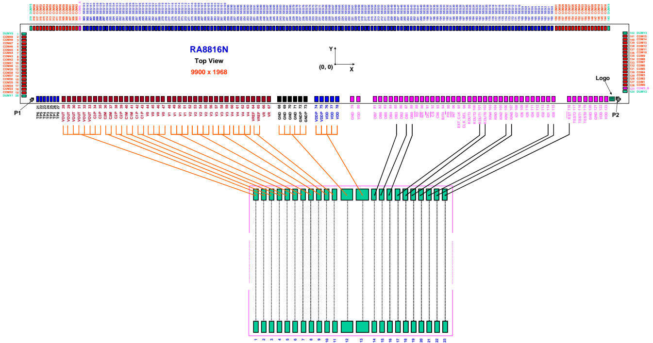
圖 A-4 : COG 模組之 FPC 接線
