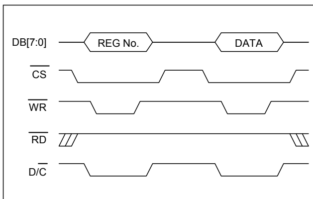
圖 6-6：以 8080 8-bit 對暫存器寫入的時序圖
