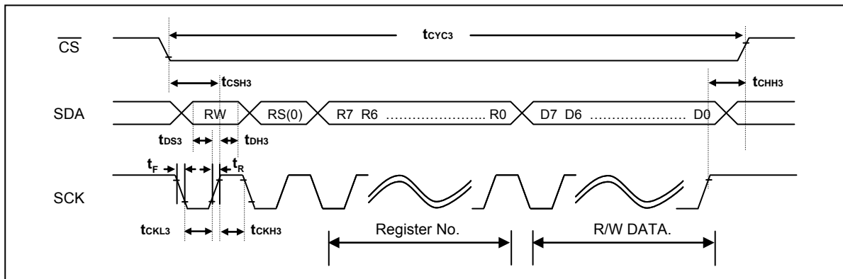
圖 9-3 : 3-Wire 時序
