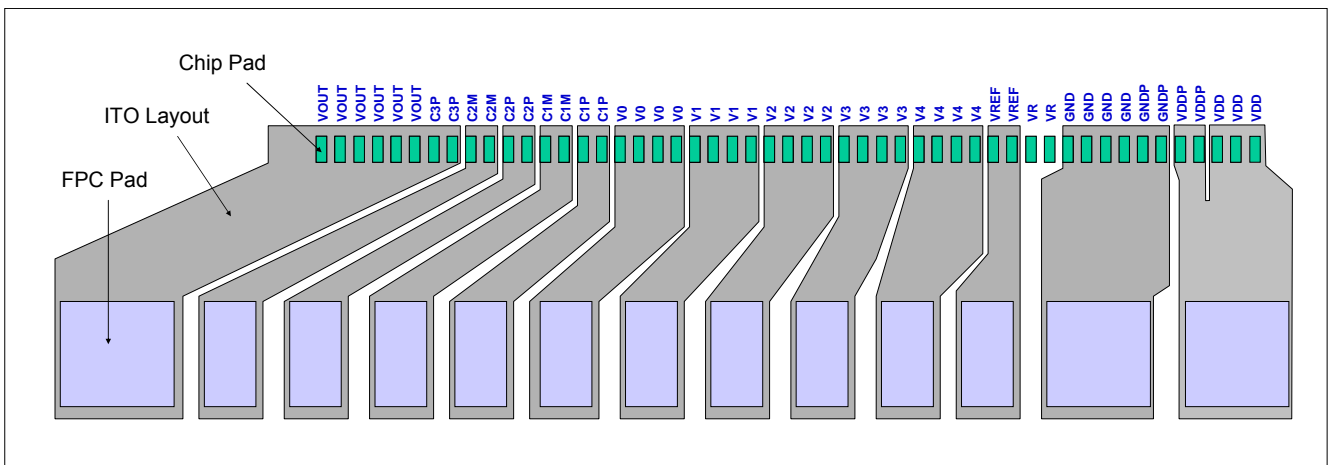
圖 A- 8：ITO 走線範例
