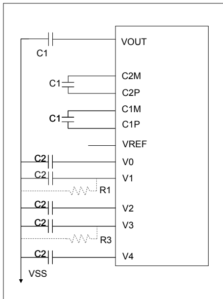
圖 6-23：使用內部 VOUT 電源電路 (3 倍壓)
