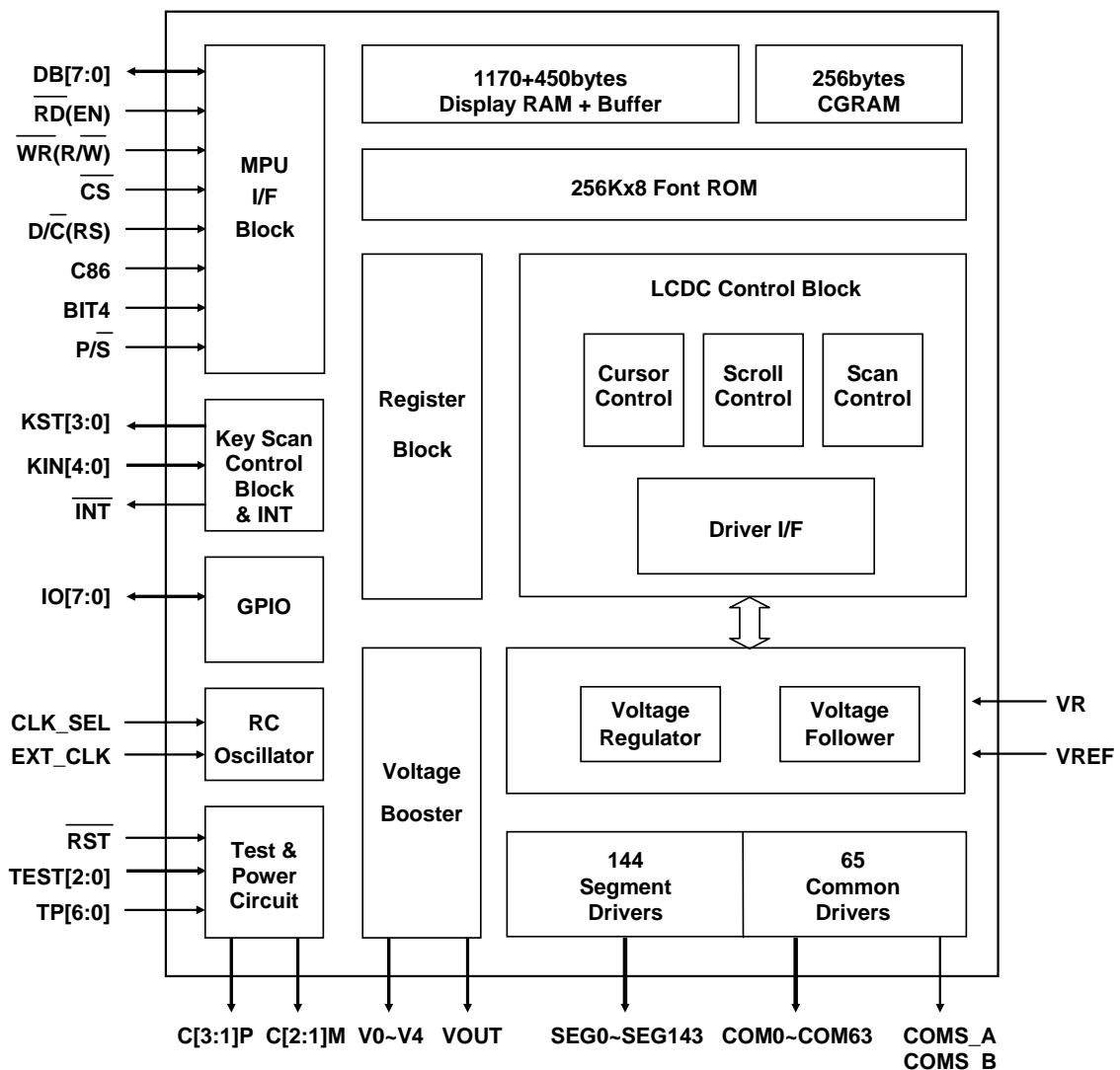
圖 3-2 : Internal Block
