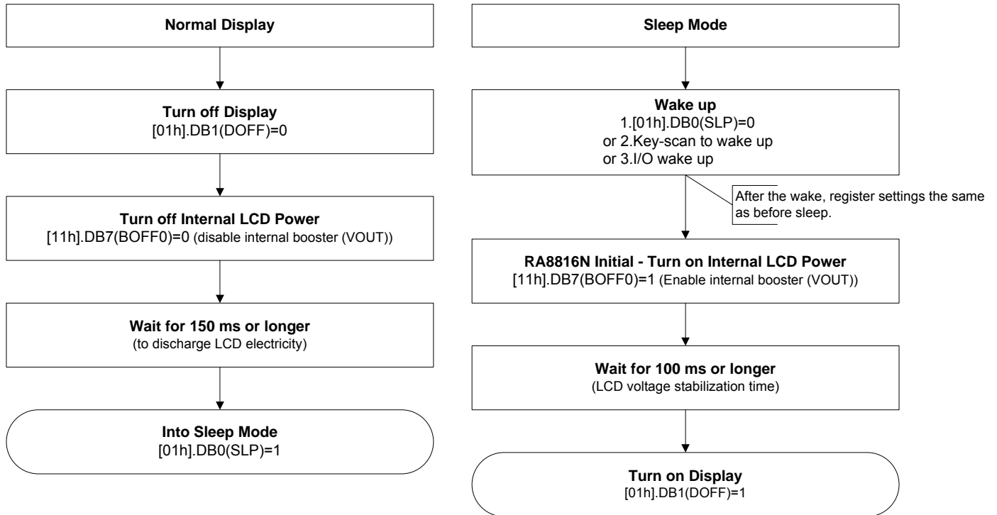
圖 6-36 : 睡眠/喚醒模式順序
