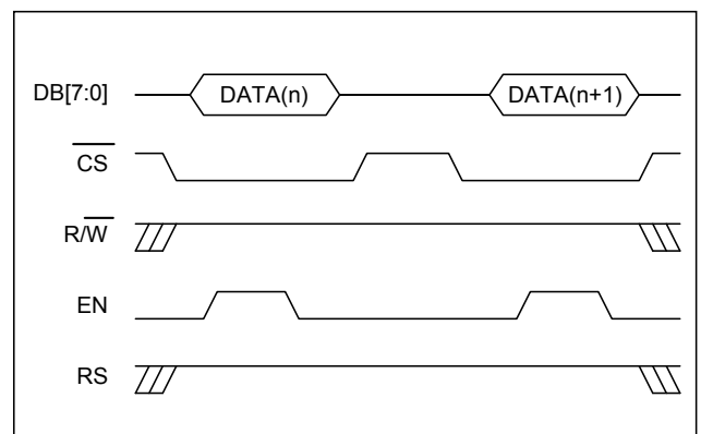
圖 6-16：以 6800 8-bit 對記憶體讀取的時序圖
