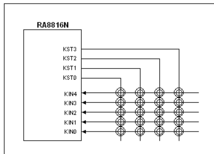
圖 6-30 : 4x5 的鍵盤掃描應用電路圖
