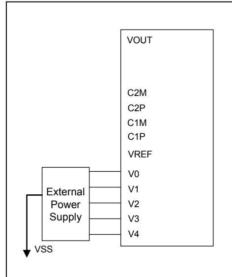
圖 6-28：使用外部分壓電源
