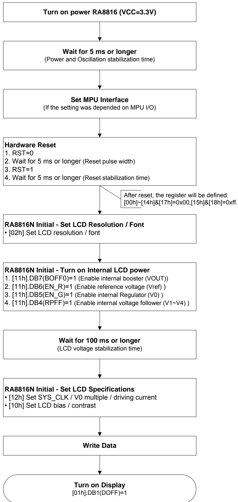
圖 6-34 : 電源開啟順序
