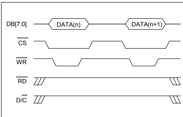
圖 6-13：以 8080 8-bit 對記憶體寫入的時序圖
