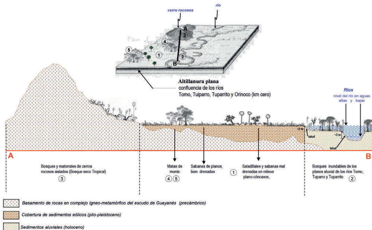
Figura 2. Perfil esquemático de los paisajes en el PNN El Tuparro, su geología y tipo de vegetación. Tomado de Villarreal (2007) y modificado.
