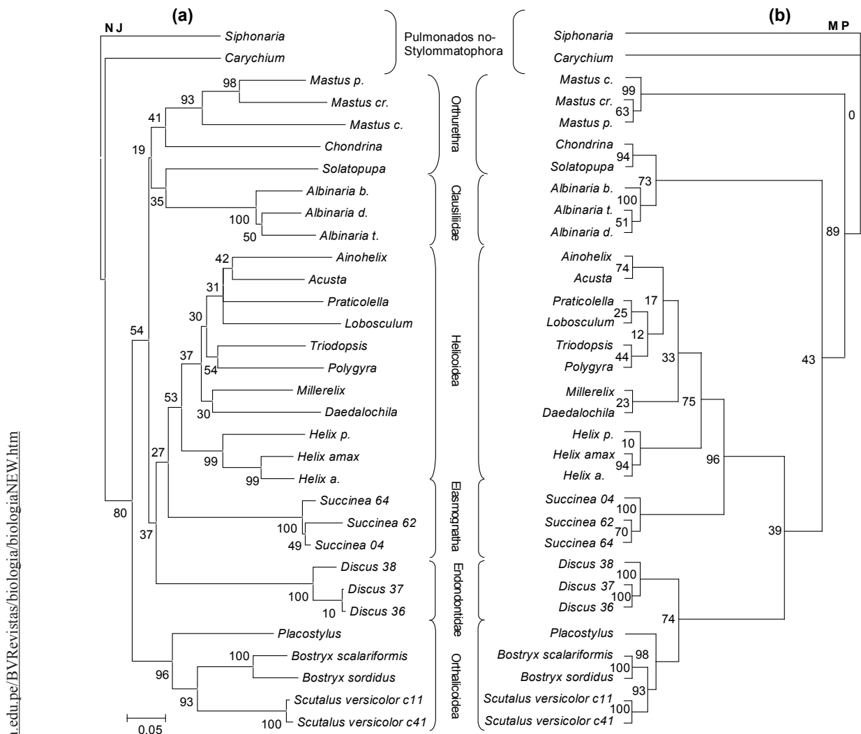
Figura 4. Árboles filogenéticos para el marcador mitocondrial 16S rRNA. (a): Topología obtenida usando NJ considerando gaps . (b): Topología obtenida usando MP considerando gaps como “nuevo estado”. Los números corresponden a valores de bootstrap . La escala corresponde al número de sustituciones por sitio. Note los altos valores de bootstrap para el grupo monofilético conformado por Bostryx y Scutalus (Familia Orthalicidae), dentro del clado de la superfamilia Orthalicoidae.
