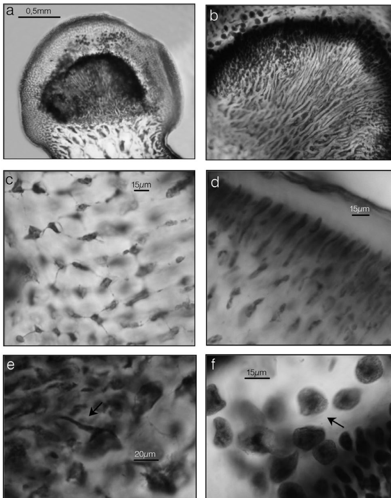
Figura 2. Cistocarpo de Hydropuntia usneoides y detalles del mismo. a: corte transversal del cistocarpo, b: gonimoblasto, c: pericarpio interno (células elongadas a estrelladas con conexiones citoplasmáticas evidentes), d: pericarpio externo (células compactas y elongadas periclinalmente), e: célula tubular nutritiva en la base del cistocarpo, f: carposporas.
