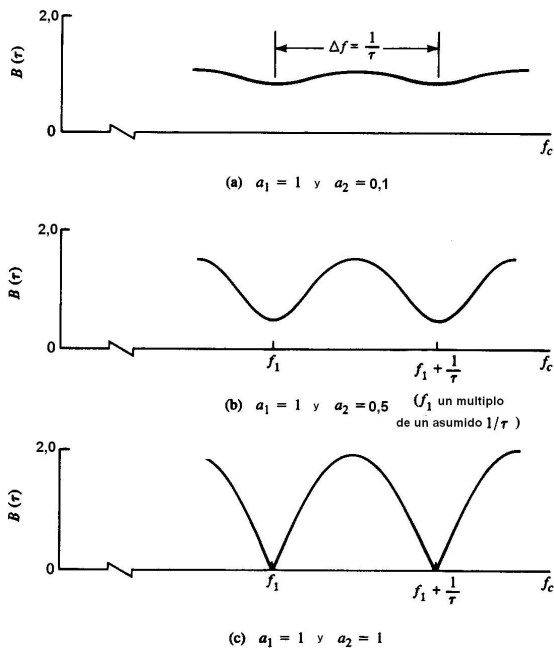
Figura 7 Graficas de B(\tau) Vs f_c
