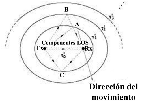
Figura 4 Modelo de propagación elíptico
