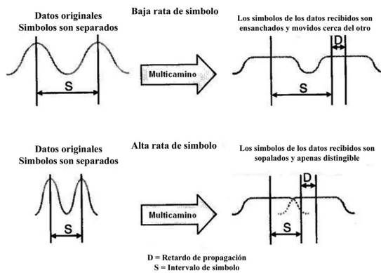
Figura 3 Interferencia Intersímbolo
