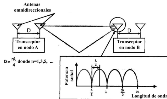
Figura 8 a) Router inalámbrico a 2,4 GHz con diversidad de antenas. b) Separación de antenas a n(\lambda/4) con n=1,3,5, \dots etc
