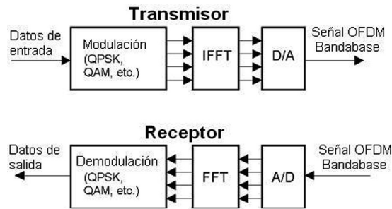
Figura 13 Sistema de comunicación basado en OFDM
