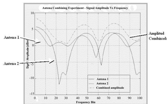
Figura 9 Potencia de recepción en un router con diversidad de dos antenas
