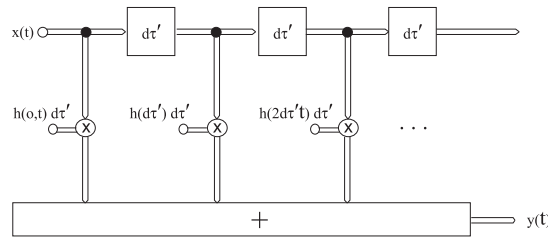
Figura 5 Representación de un canal selectivo en frecuencia
