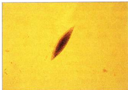
Figura 4. Microfotografía de una colonia de F. succinogenes lenticular biconvexa vista lateral (12X)
