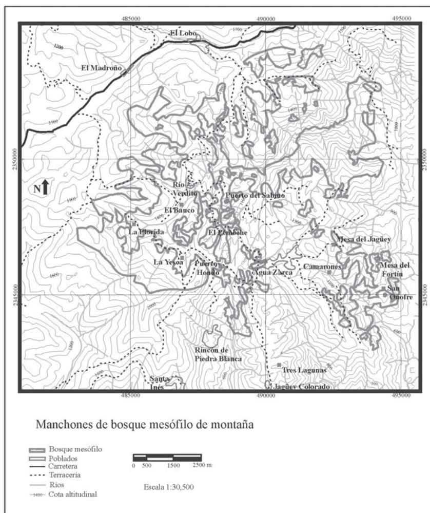
Figura 2. Mapa topográfico donde se muestran los principales manchones de bosque mesófilo de montaña de Landa de Matamoros, Querétaro. Las unidades UTM en el mapa corresponden a la zona 14-N.
