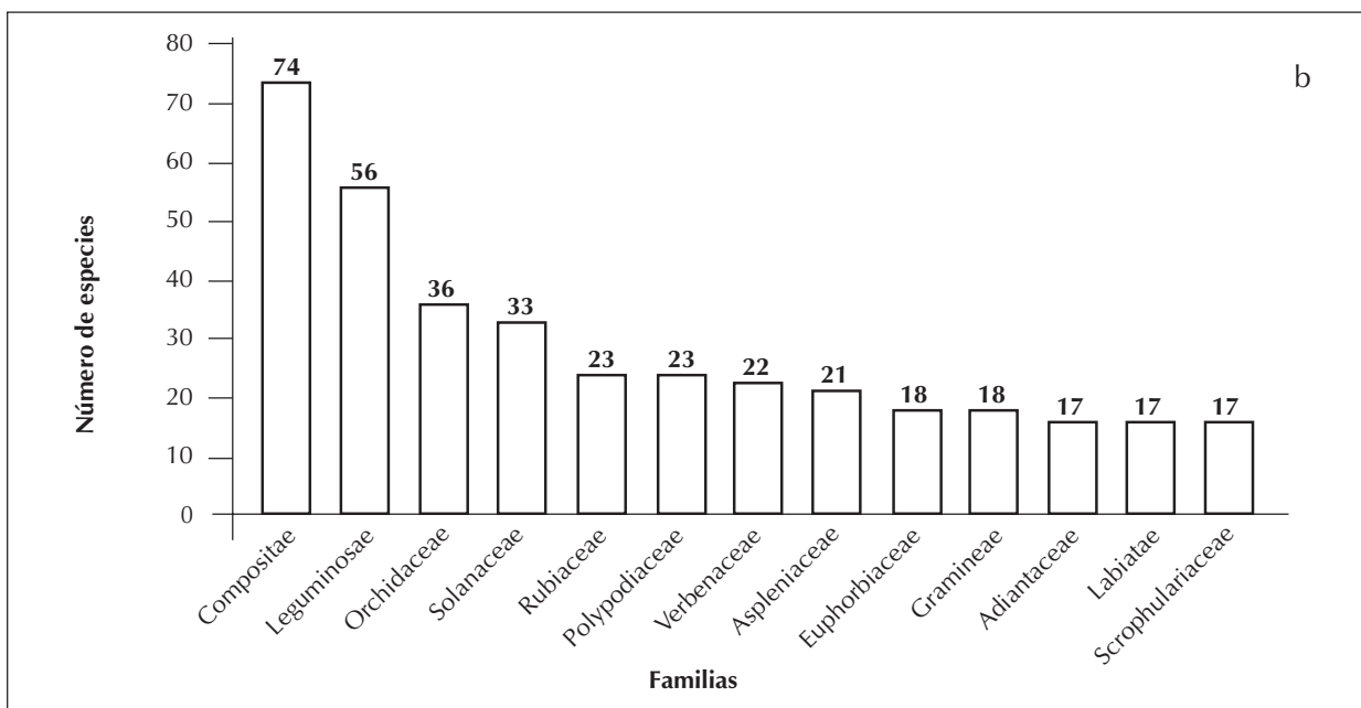
Figura 4. a) Abundancia de géneros por familia; los 258 géneros restantes pertenecen a familias variadas. b) Abundancia de especies por familia; las 400 especies restantes pertenecen a diversas familias.
