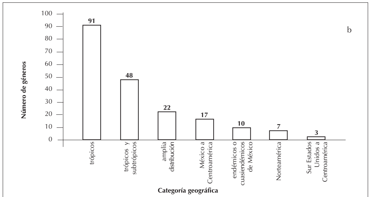
Figura 5. a) Número de especies por forma de vida. b) Distribución de los géneros presentes en Landa de Matamoros en el continente americano.
