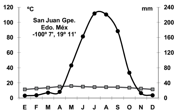
Figura 2. Diagrama ombrotérmico tipo Gausen de la región de estudio obtenido a partir de la estación San Juan Guadalupe
