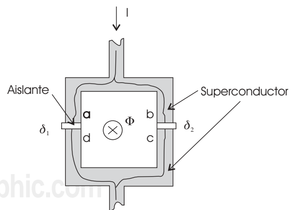
Figura 3. Uniones Josephson conectadas en paralelo. I es la corriente de alimentación, \Phi es el flujo magnético externo, \delta_1 y \delta_2 son las diferencias de fase de la corriente a través de las uniones.
