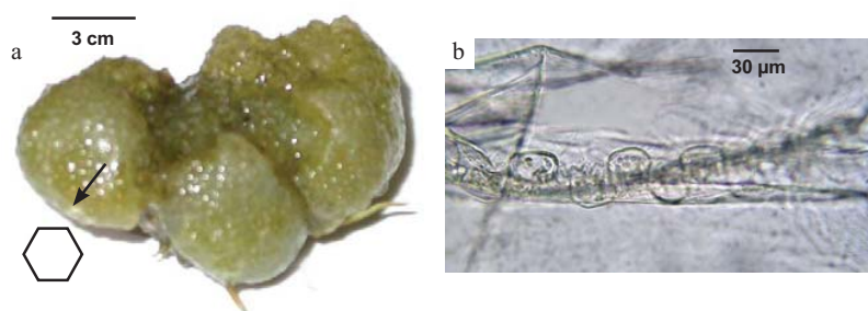
Fig. 5. Dictyosphaeria cavernosa . a. Hábito. b. Células hapteroidales.
