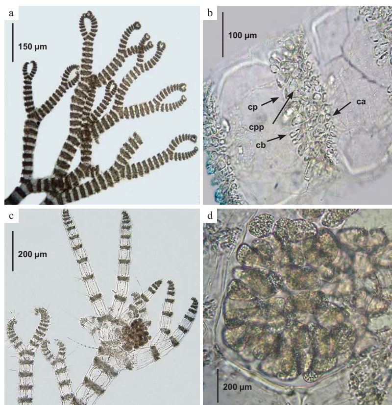
Fig. 9. Ceramium clarionense . a. Hábito. b. Detalle de las células del nudo. c. Rama con estructura reproductiva. d. Detalle de un gonimocarpo. ca = células acrópetas, cb = células basípetas, cp = células periaxiales, cpp = células pseudoperiaxiales.
