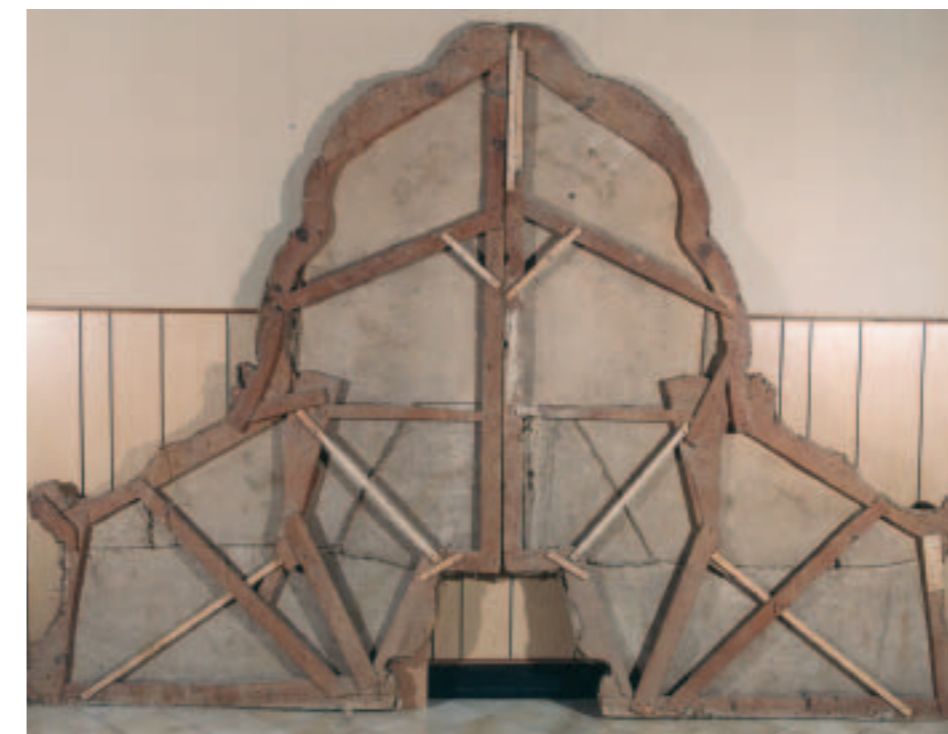
4. Il telaio ligneo della "veletta", prima del restauro.
